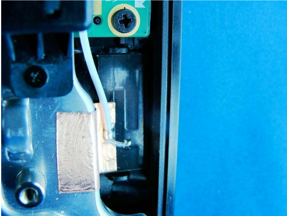
(19) EUT Photo (Antenna-Aux)
