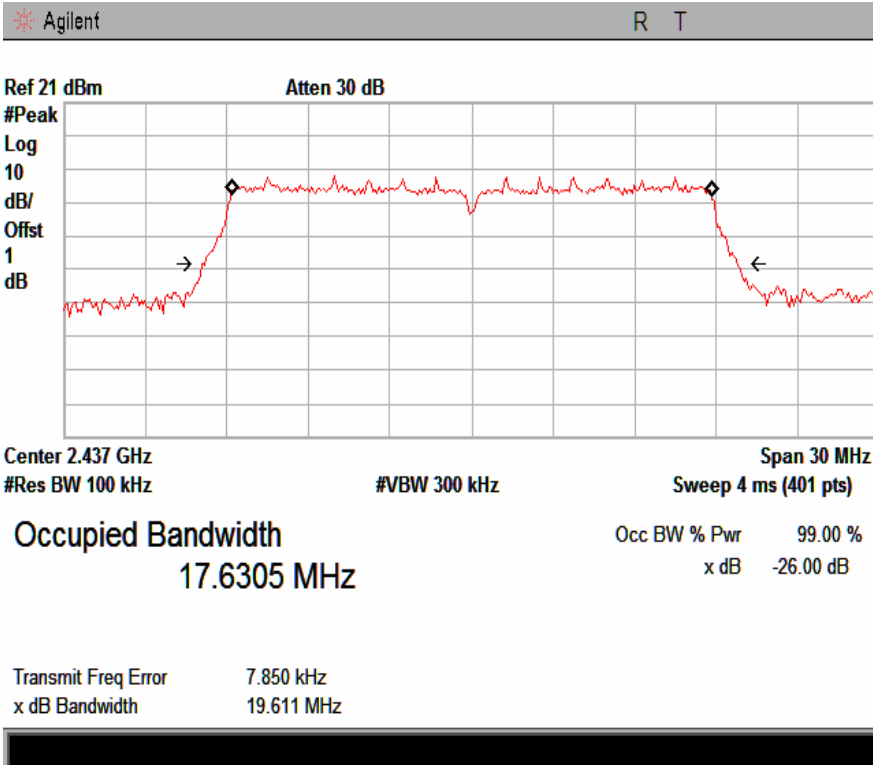
802.11n-26dB-mid
