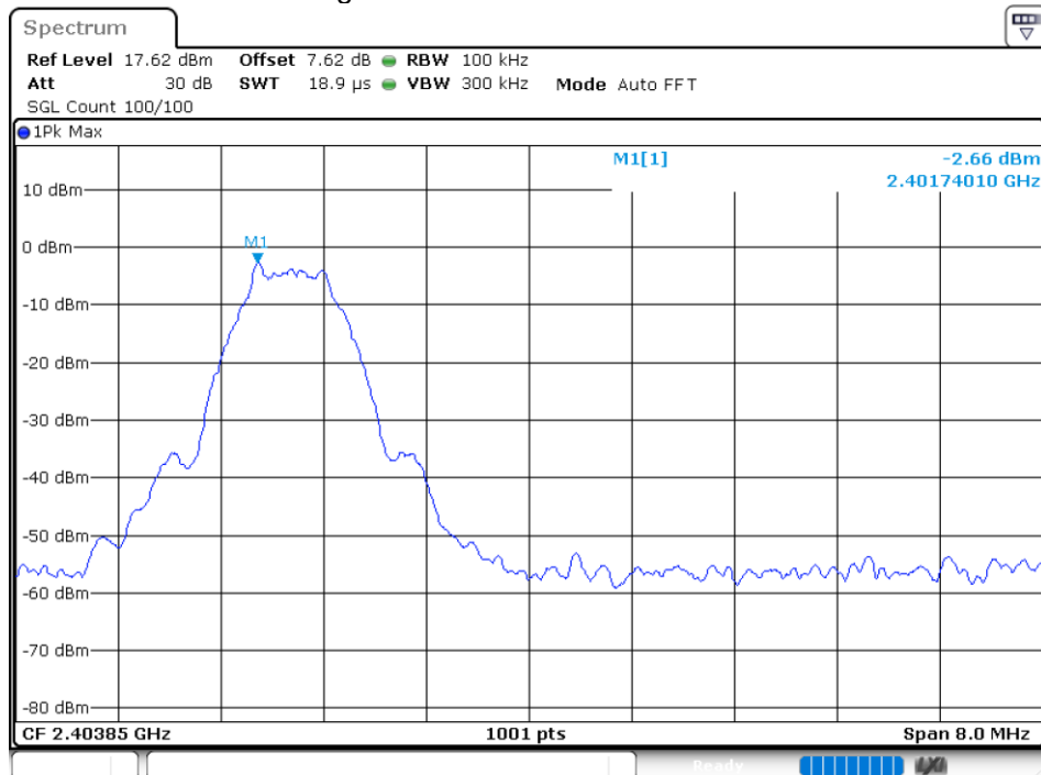
Band Edge NVNT BLE 2403.85MHz Ant1 Ref
