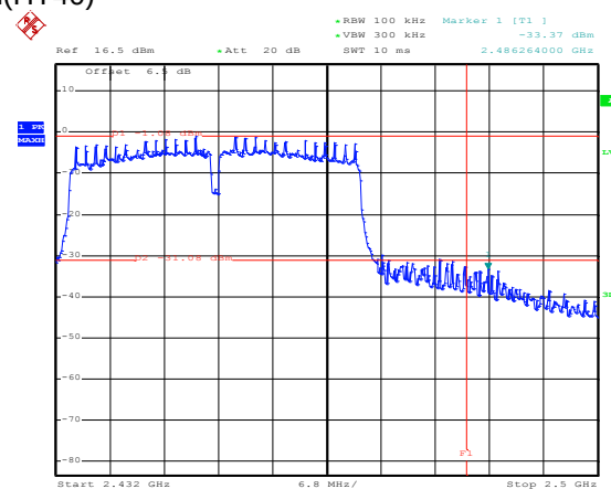
802.11n(HT40)
