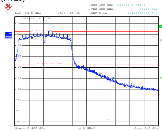
802.11n(HT20)
