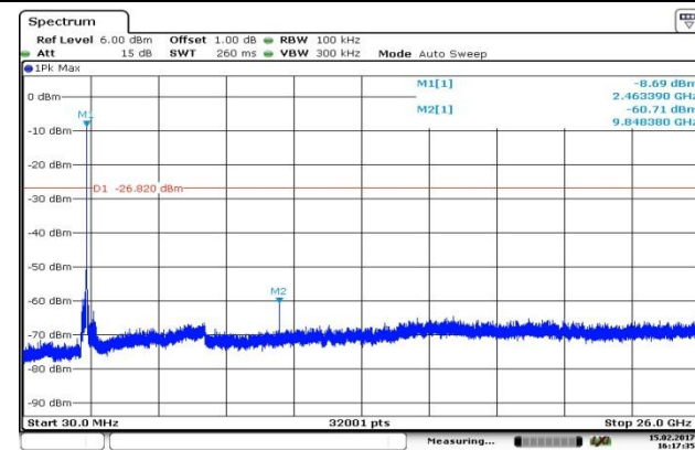
CH11-SE
