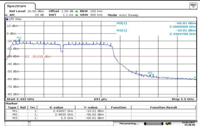
CH09-Bandedge
