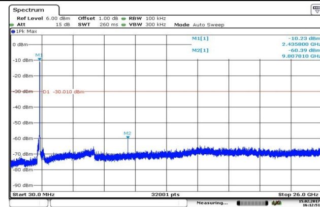
CH09-SE
