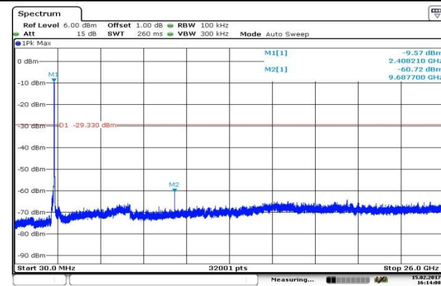
CH03-SE
