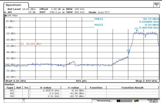
CH01-Bandedge
