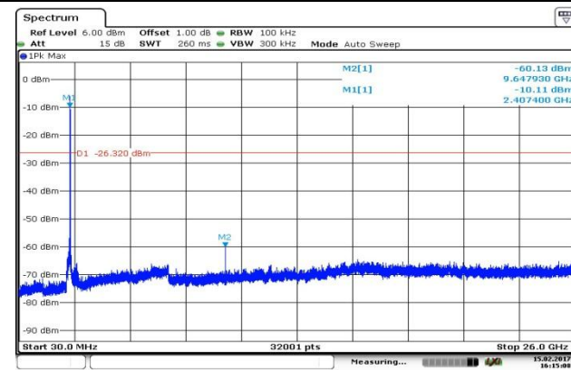
CH01-SE
