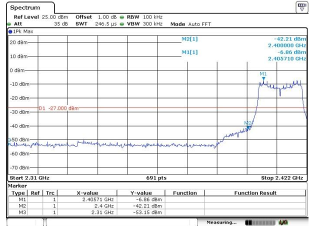
CH01-Bandedge
