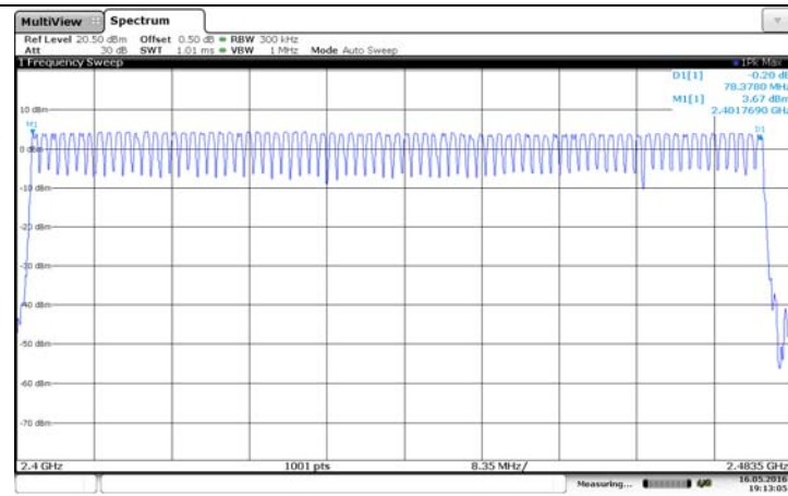
GFSK
