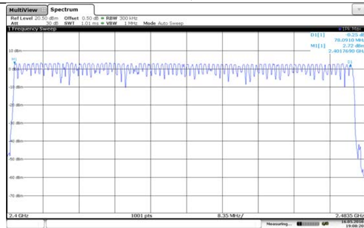
8DPSK
