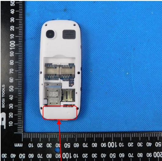
GSM ANT
