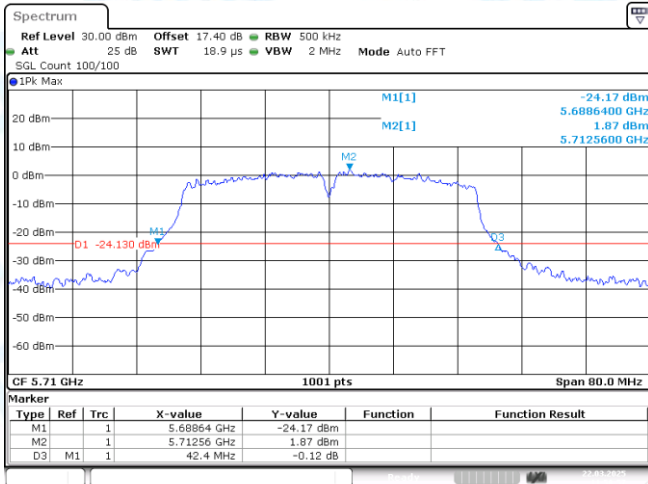
11AX40MIMO-Ant1-5710
