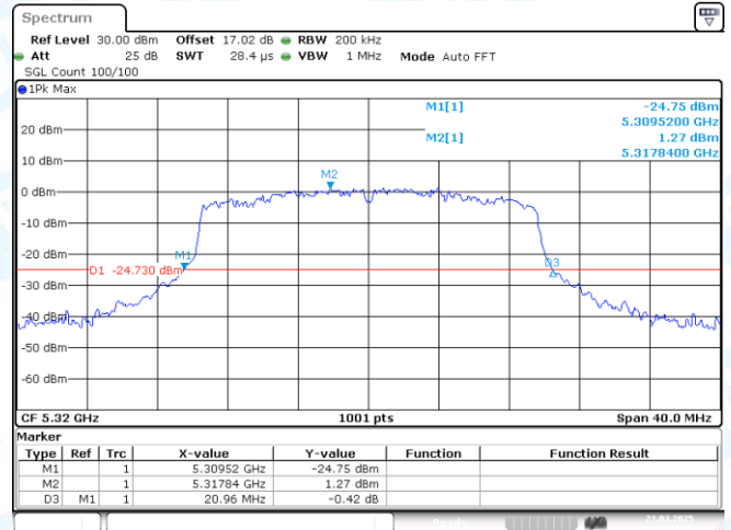
11AX20MIMO-Ant2-5320
