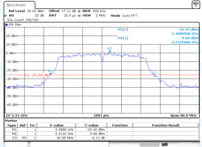
11AX40MIMO-Ant2-5510
