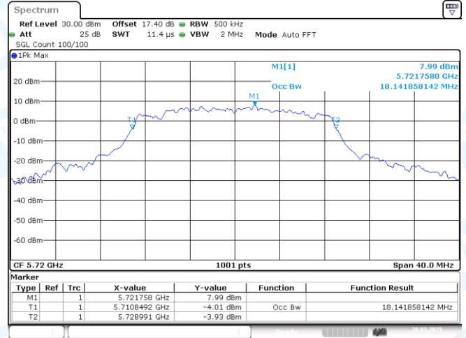
11N20MIMO-Ant1-5720
