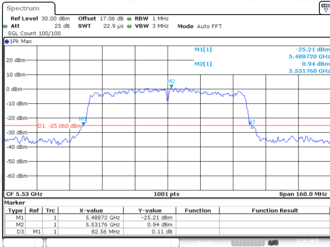
11AX80MIMO-Ant1-5530
