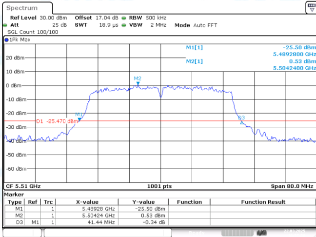
11AX40MIMO-Ant1-5510
