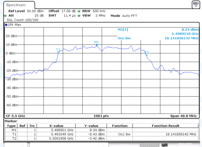
11N20MIMO-Ant1-5500
