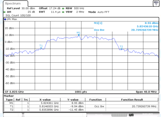
11N20MIMO-Ant1-5825
