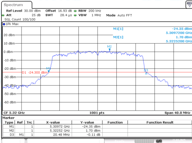
11AX20MIMO-Ant1-5320
