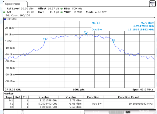
11N20MIMO-Ant1-5260
