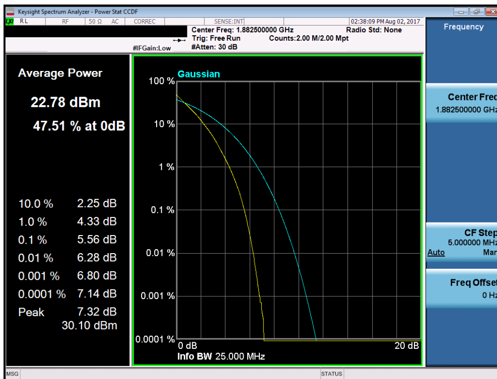
Plot 7-192. PAR Plot (Band 2/25 – 20.0MHz QPSK – RB Size 100)
