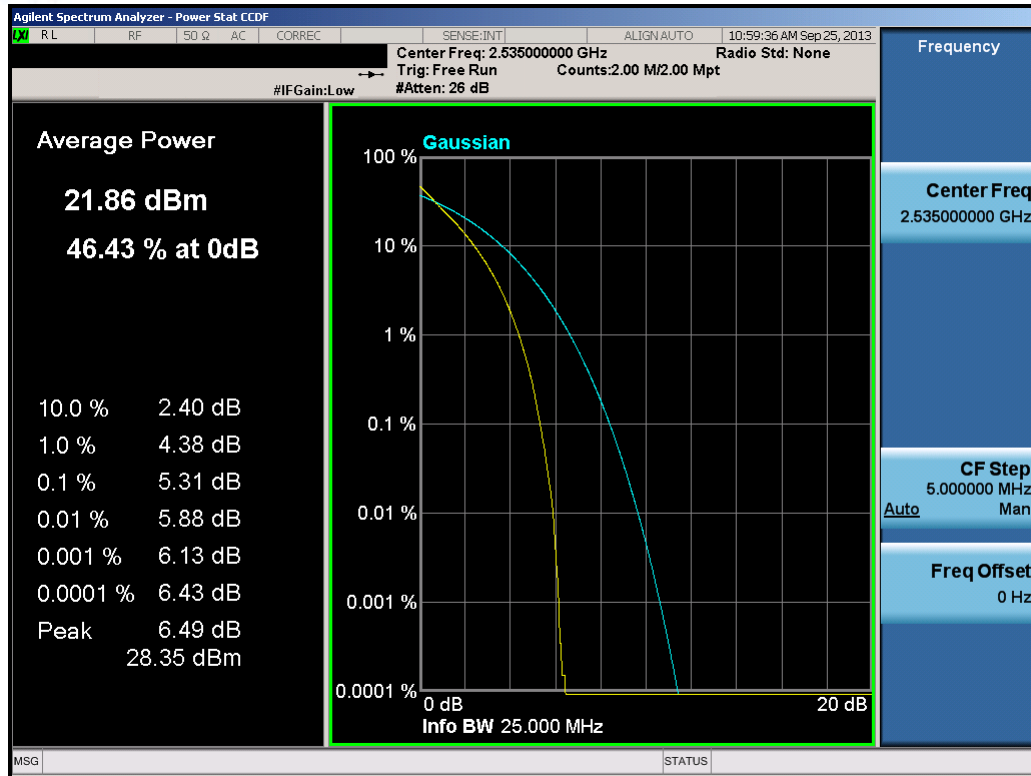
Plot 11-46. PAR Plot (20.0MHz QPSK – RB Size 100)
