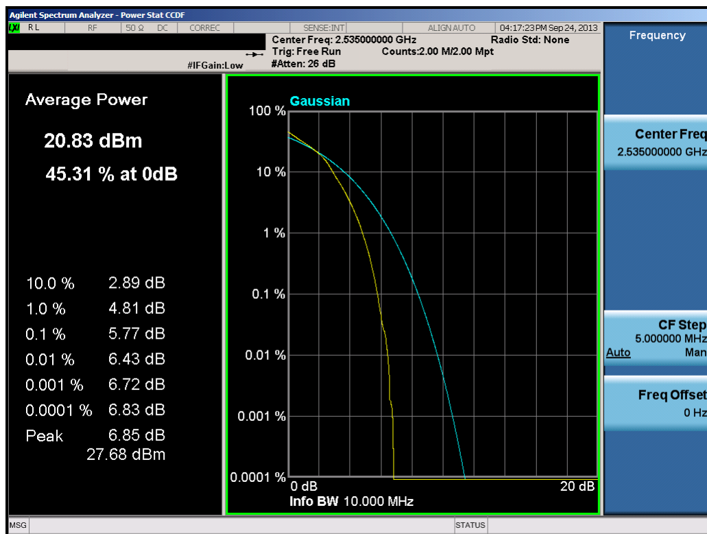
Plot 11-25. PAR Plot (10.0MHz 16-QAM – RB Size 50)
