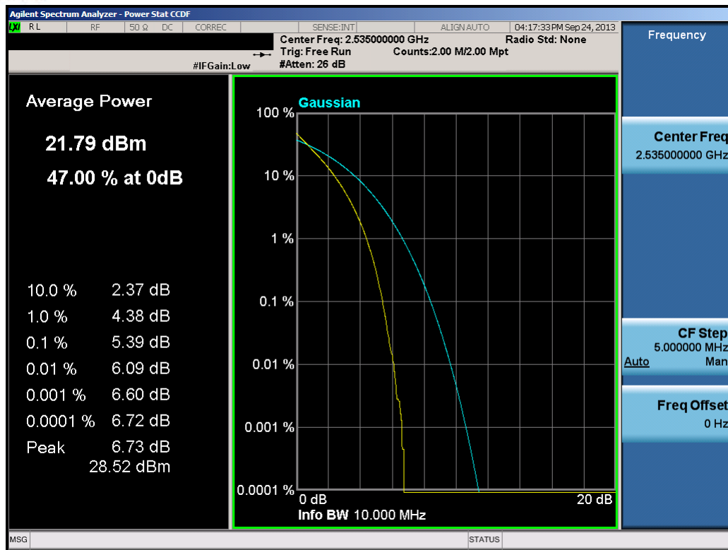
Plot 11-24. PAR Plot (10.0MHz QPSK – RB Size 50)
