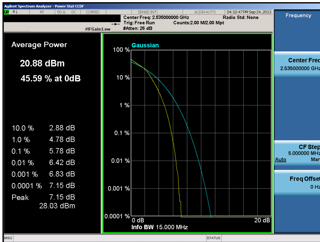
Plot 11-36. PAR Plot (15.0MHz 16-QAM – RB Size 75)
