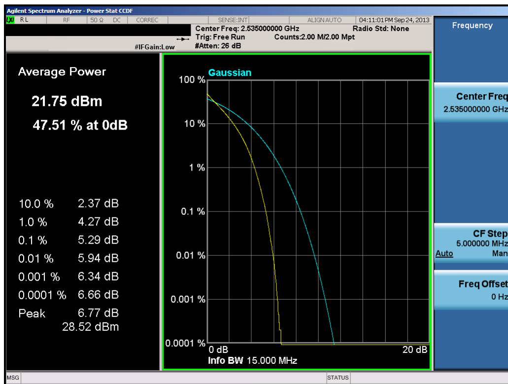
Plot 11-35. PAR Plot (15.0MHz QPSK – RB Size 75)
