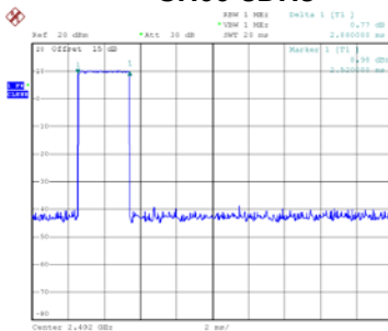
CH00-3DH5
