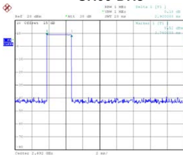
CH00-DH5
