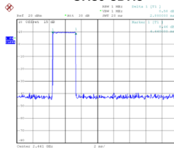
CH39-3DH5
