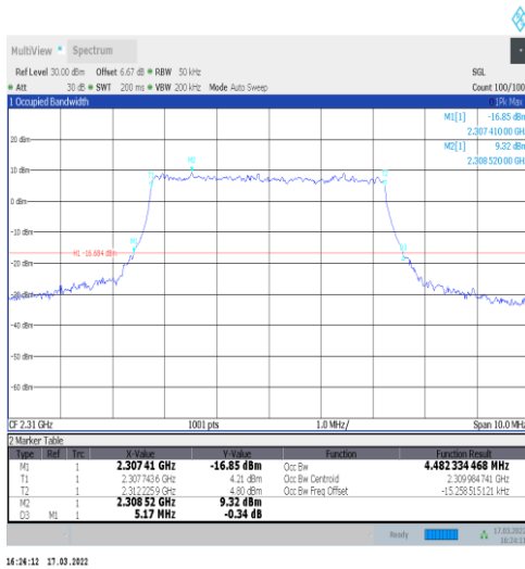
1-N30-15-5-M-6-CP-QPSK-Outer_Full-25@0-Ant1-4. 482-5.170-≤5-PASS
