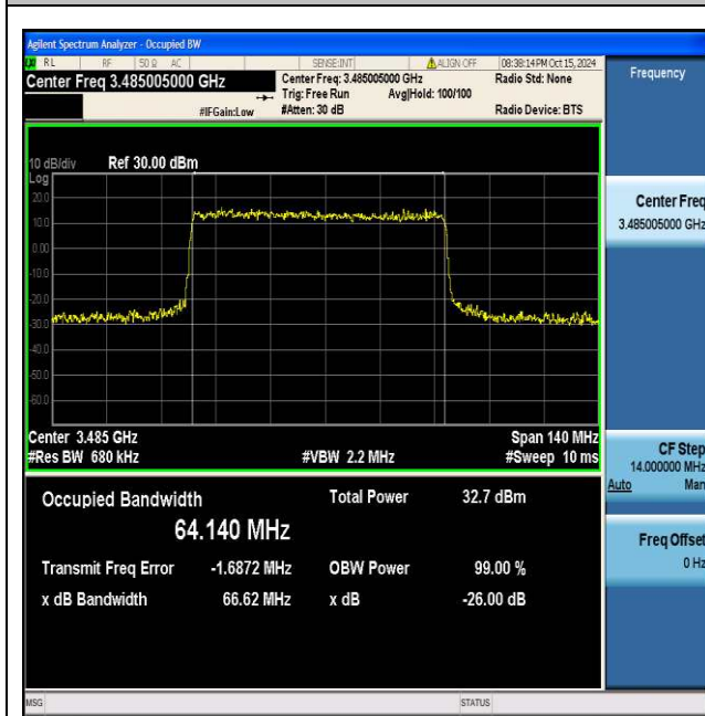
NTNV_N77-3450-3550_PC2_30_70_L_TID3_Ant1#1
