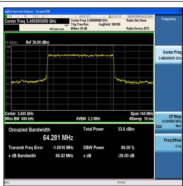
NTNV_N77-3450-3550_PC2_30_70_L_TID2_Ant1#1
