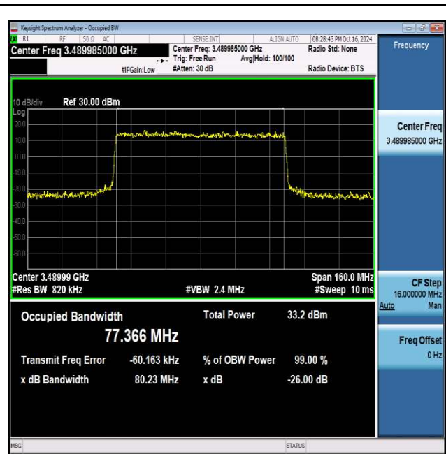
NTNV_N77-3450-3550_PC2_30_80_L_TID6_Ant1#1
