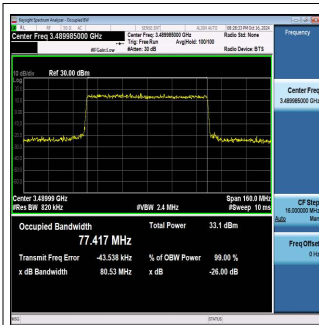
NTNV_N77-3450-3550_PC2_30_80_L_TID5_Ant1#1
