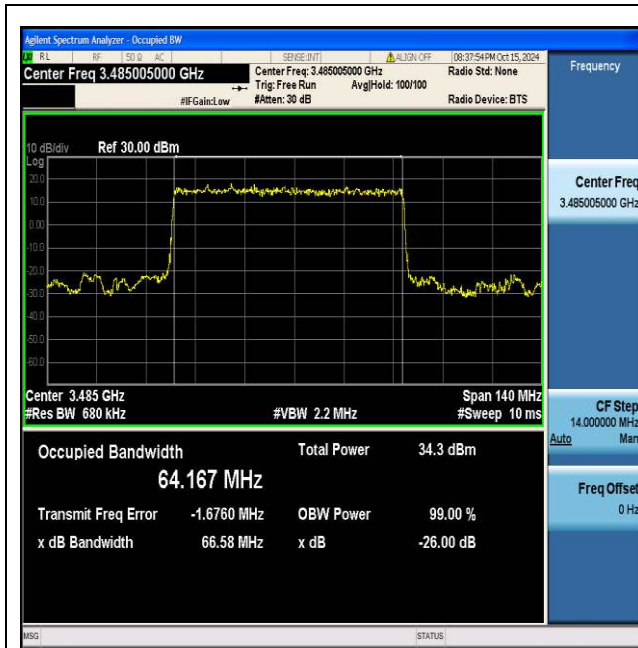
NTNV_N77-3450-3550_PC2_30_70_L_TID1_Ant1#1
