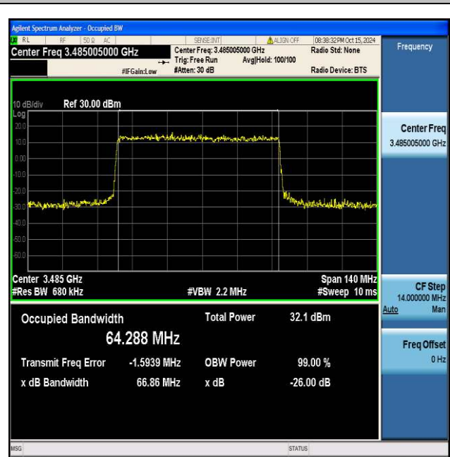
NTNV_N77-3450-3550_PC2_30_70_L_TID4_Ant1#1
