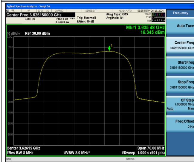
48-48-20MHz-15MHz-QPSK-QPSK-55916-56087-100RB#0- 75RB#0-PASS
