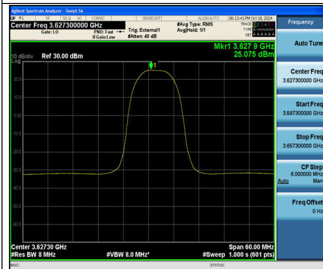
48-48-20MHz-10MHz-QPSK-QPSK-55941-56085-1RB#99- 0RB#0-PASS
