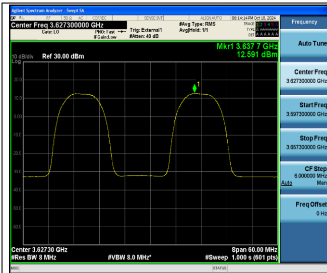
48-48-20MHz-10MHz-QPSK-QPSK-55941-56085-1RB#0- 1RB#49-PASS
