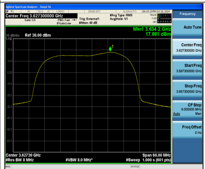
48-48-20MHz-10MHz-QPSK-QPSK-55941-56085-100RB#0- 50RB#0-PASS
