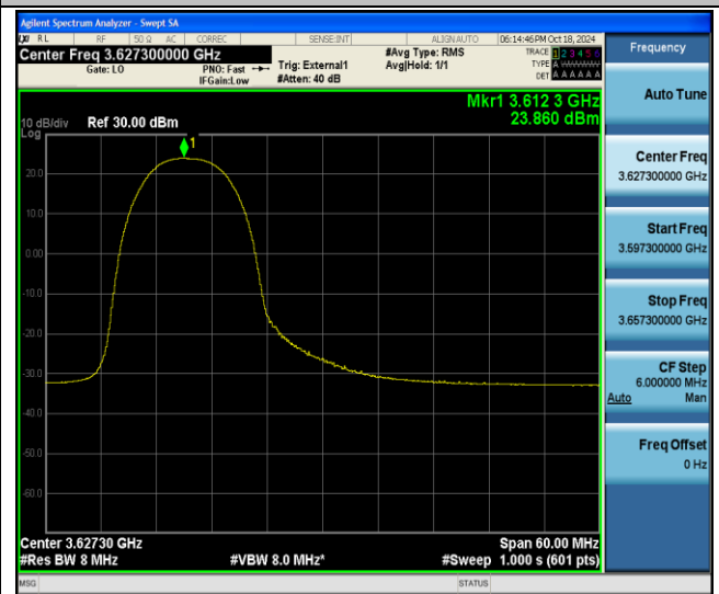
48-48-20MHz-10MHz-QPSK-QPSK-55941-56085-18RB#0- 0RB#0-PASS
