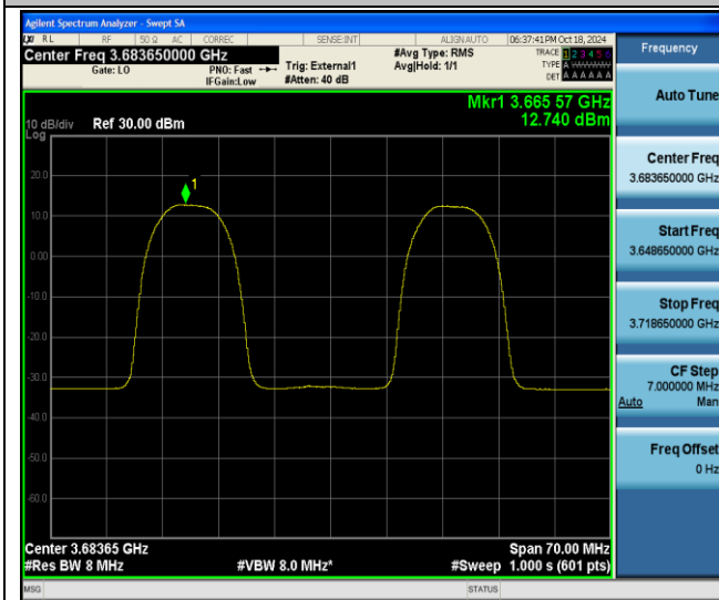
48-48-20MHz-15MHz-QPSK-QPSK-56491-56662-1RB#0- 1RB#74-PASS
