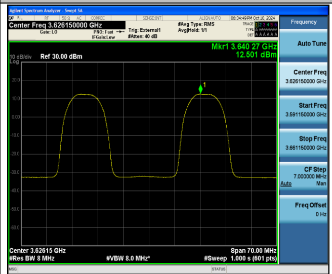
48-48-20MHz-15MHz-QPSK-QPSK-55916-56087-1RB#0- 1RB#74-PASS
