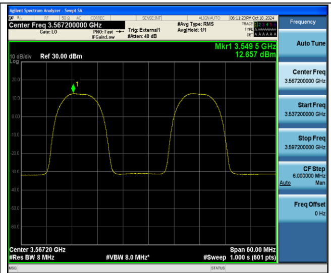
48-48-20MHz-10MHz-QPSK-QPSK-55340-55484-1RB#0- 1RB#49-PASS
