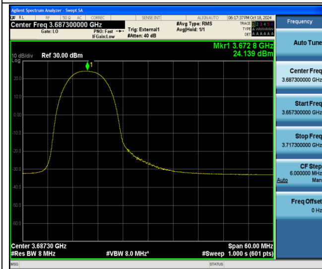
48-48-20MHz-10MHz-QPSK-QPSK-56541-56685-18RB#0- ORB#0-PASS
