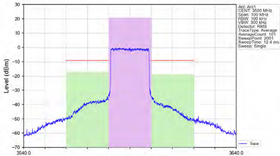
Band42c_20MHz_QPSK_HCH_3590MHz_RB_100_0_NTNV
