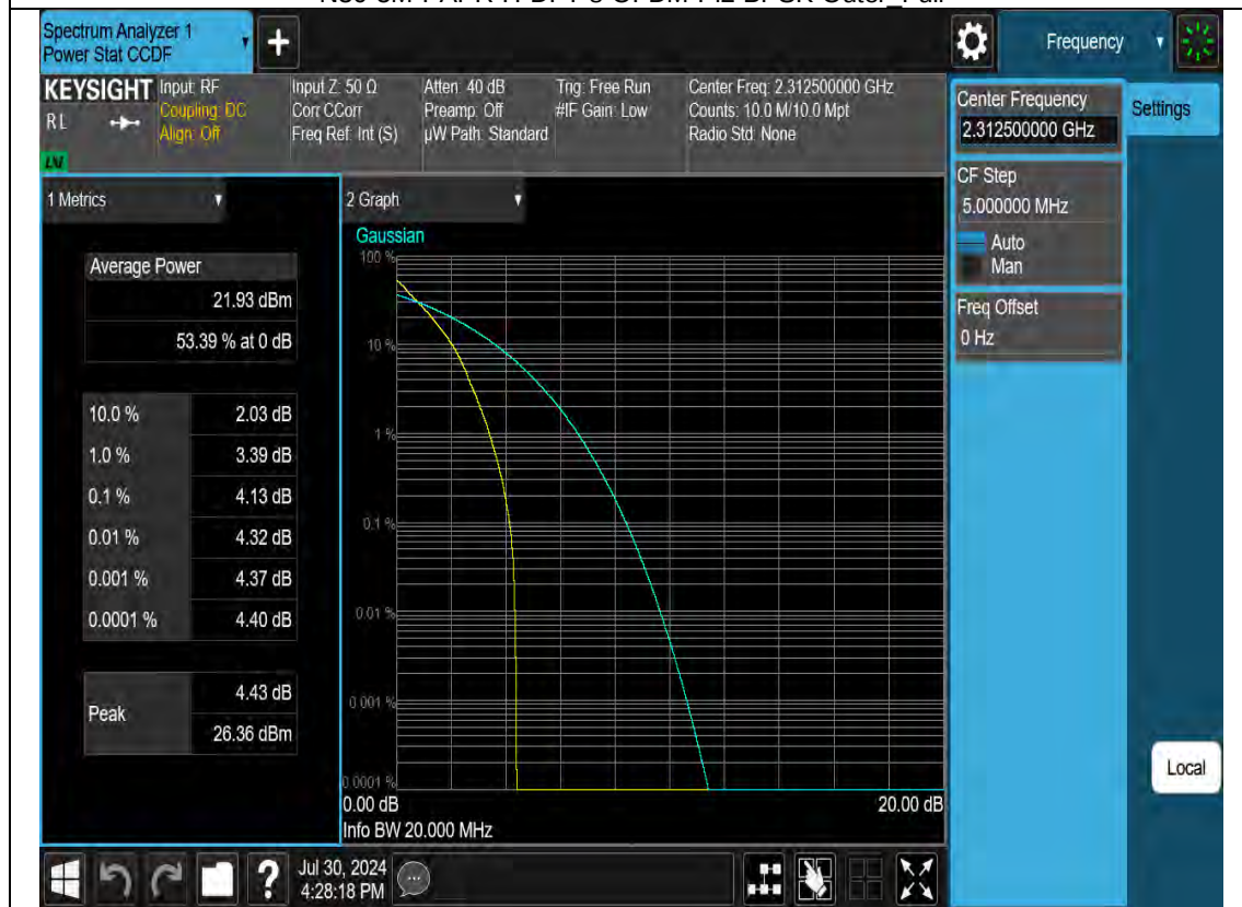
N30-5M-PAPR-H-CP-OFDM-QPSK-Outer_Full
