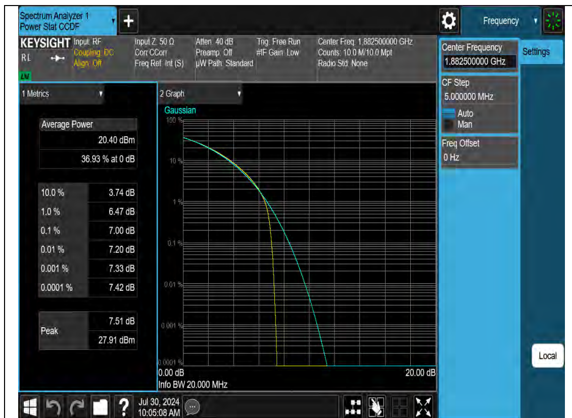
N25-20M-PAPR-H-DFT-s-OFDM-Pi2 BPSK-Outter Full
