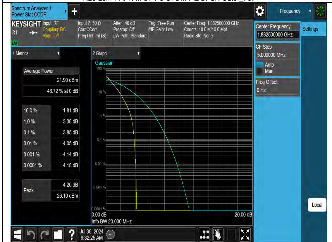
N25-20M-PAPR-M-CP-OFDM-QPSK-Outer Full
