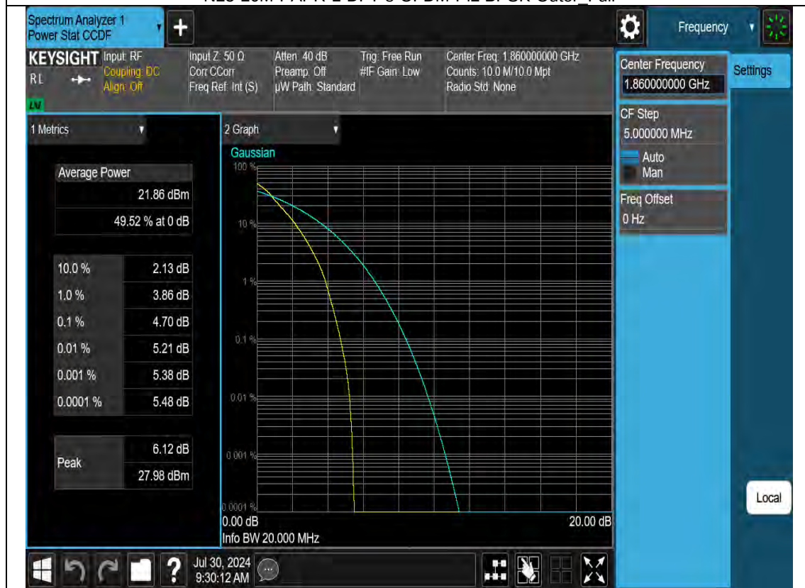
N25-20M-PAPR-L-CP-OFDM-QPSK-Outer Full
