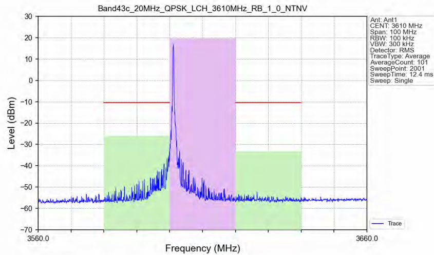
Band43c 20MHz QPSK LCH 3610MHz RB 1 0 NTNV
