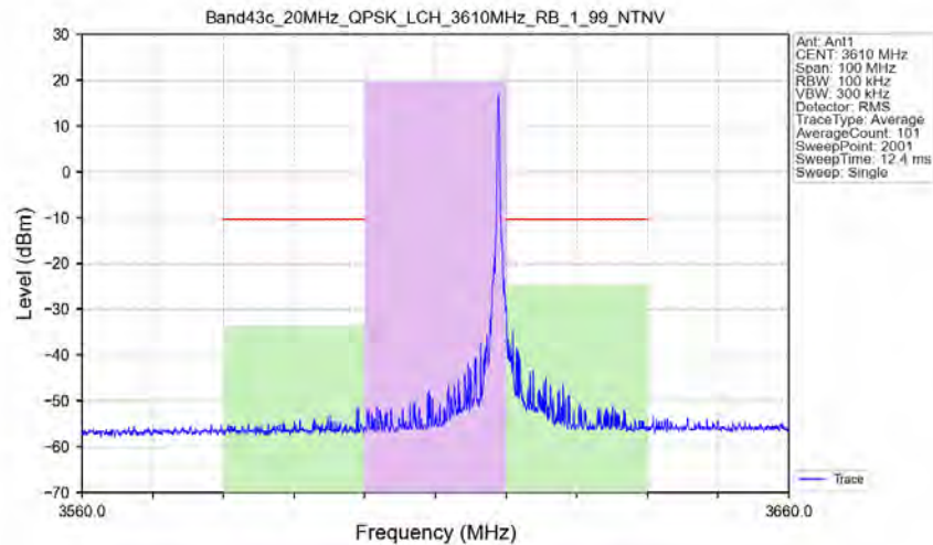
Band43c 20MHz QPSK LCH 3610MHz RB 1 99 NTNV
