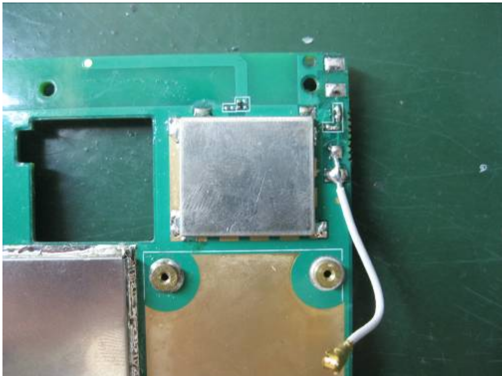
WiFi Module
