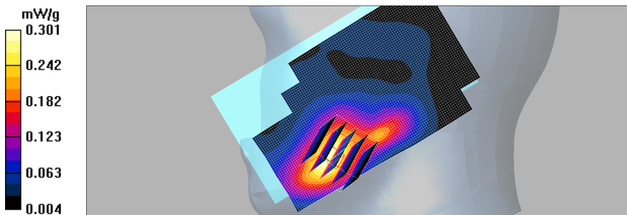
Fig.7 WCDMA1900 CH9538
