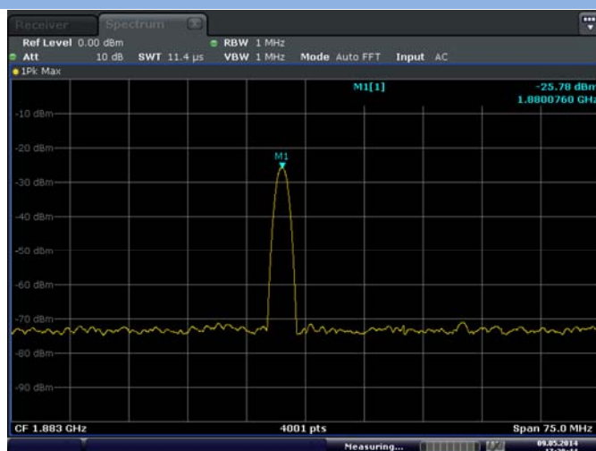
A.6.5 GSM 1900MHz CHANNEL 661
