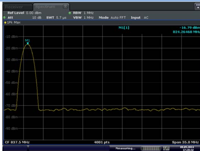
A.6.1 GSM 850MHz CHANNEL 128
