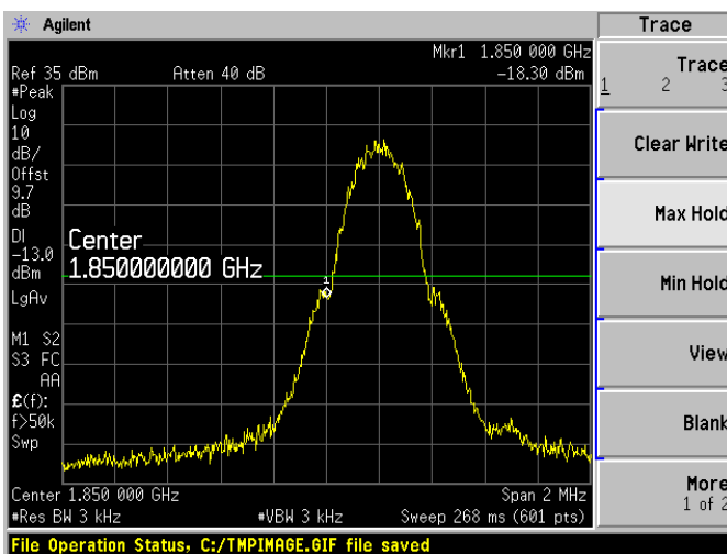
A.5.3 GSM 1900MHz CHANNEL 512
