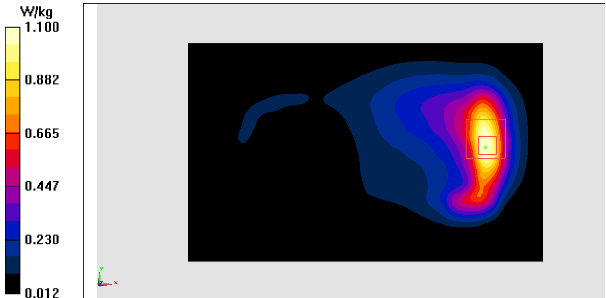
Fig.14 LTE Band4
