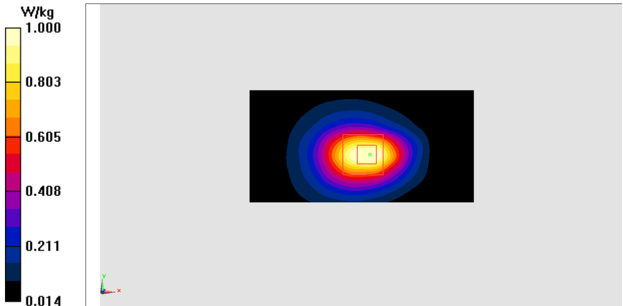
Fig.12 LTE Band2
