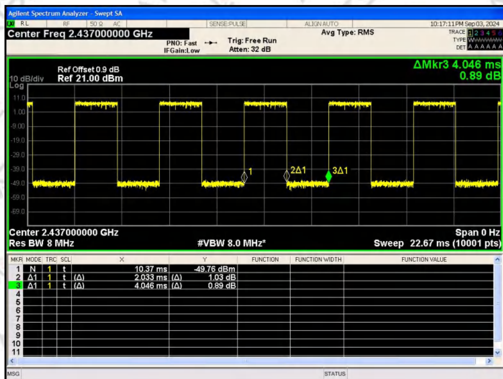
IEEE 802.11g_20MHz_Channel 6
