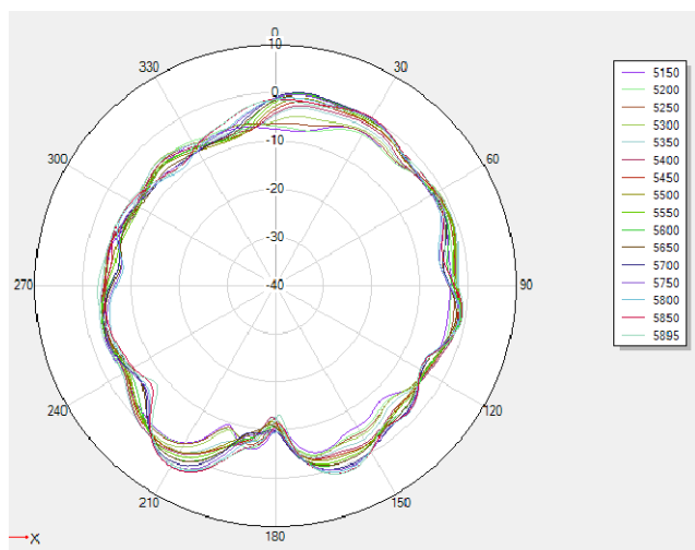
5G phi=0deg
