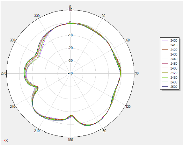
2.4G phi=0deg
