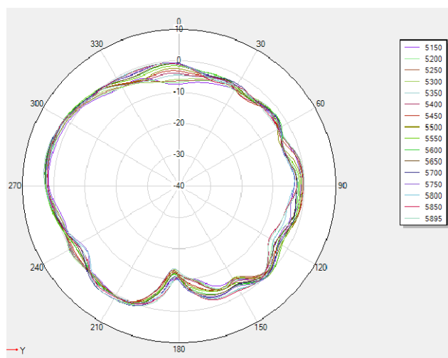
5G phi=90deg
