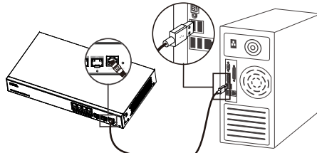
Anbindung über den Konsole-Port (USB)
