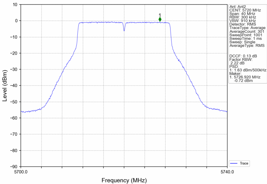
802.11n(HT20)_HCH_5720MHz_Ant2_NTNV
