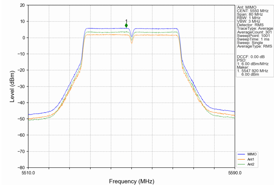
802.11n(HT40)_MCH_5550MHz_MIMO_NTNV
