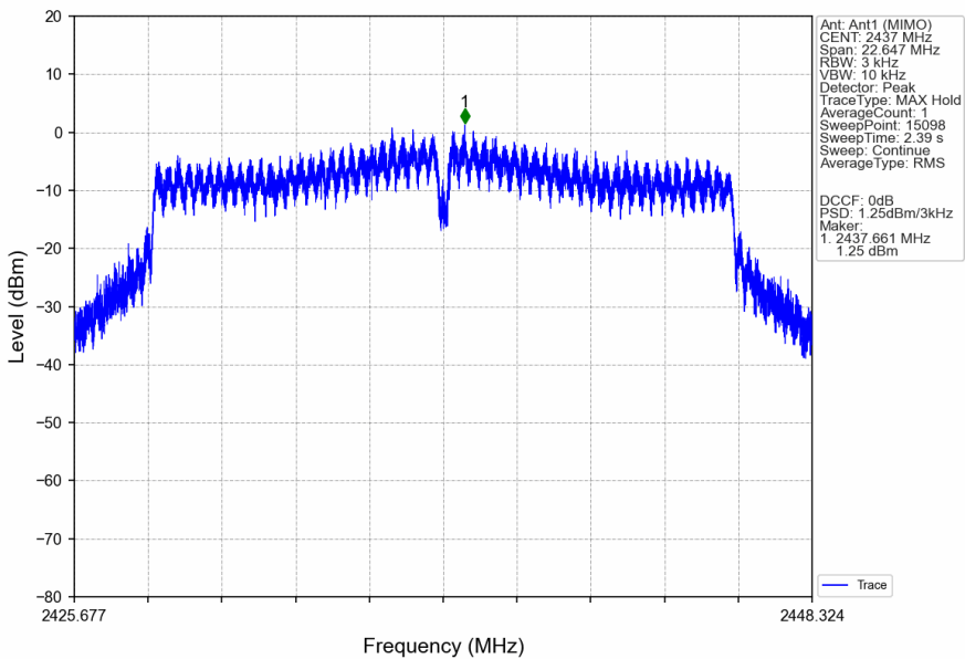
802.11n(HT20)_MCH_2437MHz_Ant1 (MIMO)_NTNV
