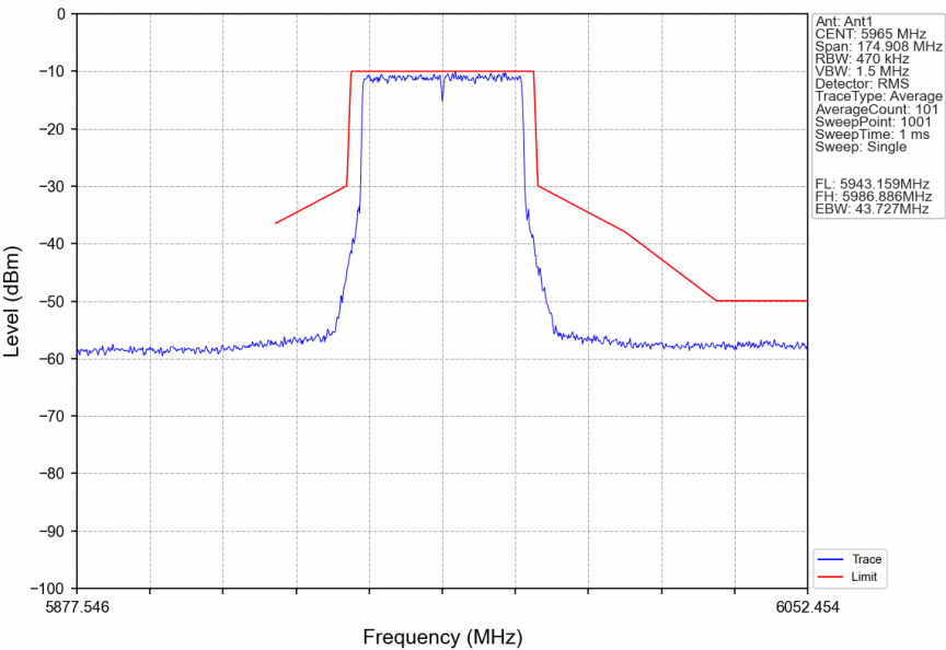
802.11ax(HEW40)_LCH_5965MHz_RU484_Left_Ant1_NTNV
