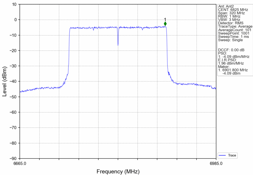
802.11ax(HEW160)_HCH_6825MHz_2xRU996_Left_Ant2_NTNV
