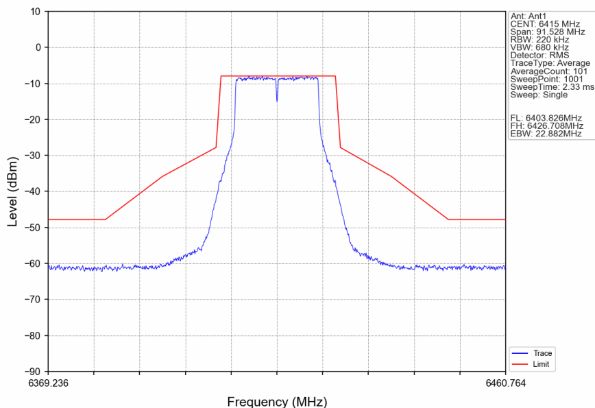
802.11a_HCH_6415MHz_Ant1_NTNV
