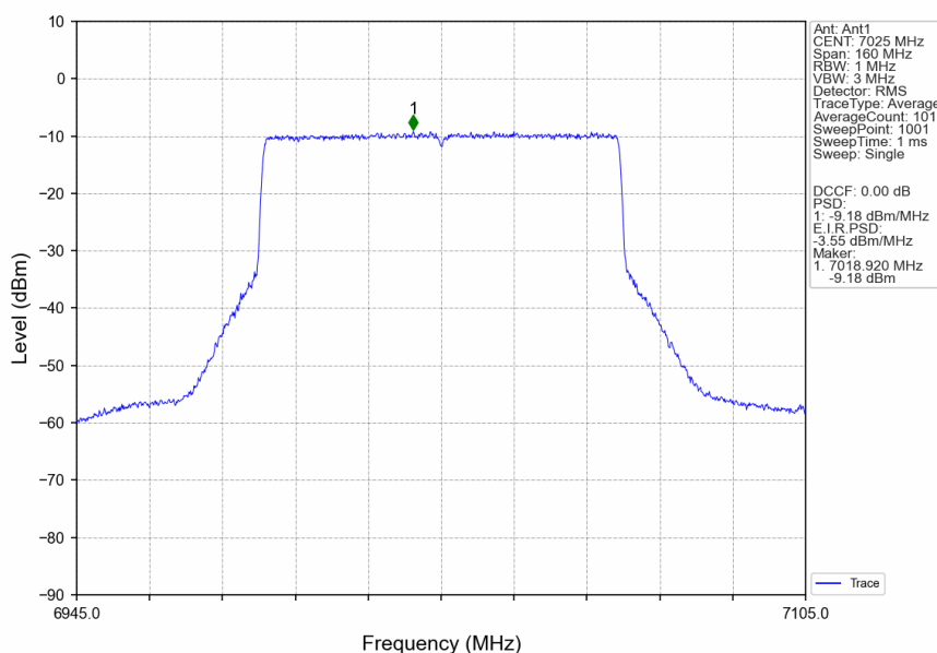
802.11ax(HEW80)_HCH_7025MHz_RU996_Left_Ant1_NTNV
