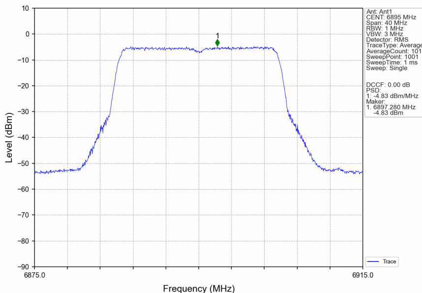
802.11ax(HEW20)_LCH_6895MHz_RU242_Left_Ant1_NTNV
