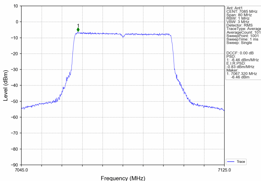
802.11ax(HEW40)_HCH_7085MHz_RU484_Left_Ant1_NTNV
