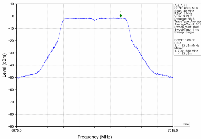
802.11a_MCH_6995MHz_Ant1_NTNV
