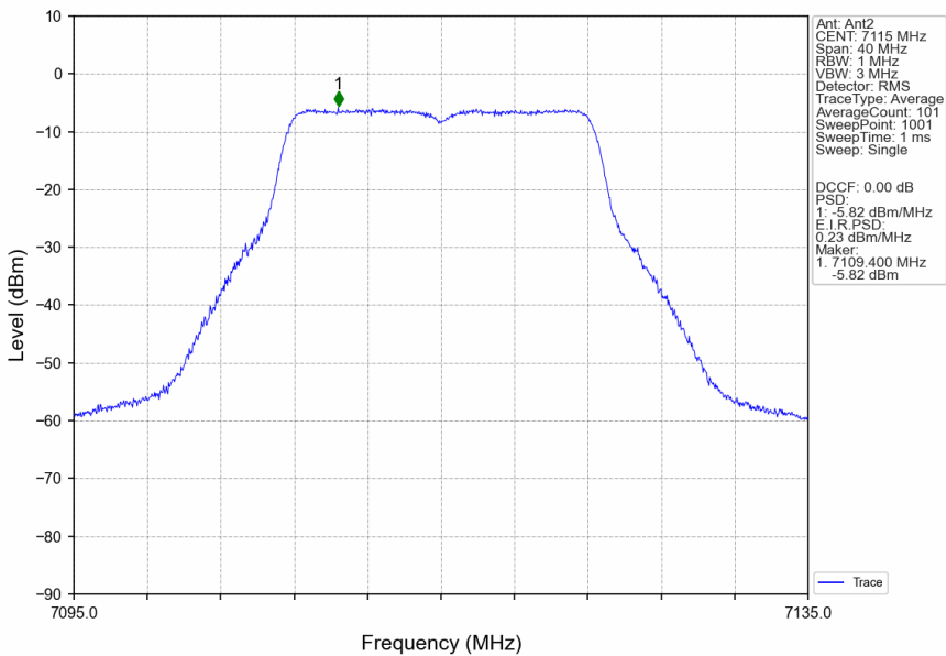
802.11a_HCH_7115MHz_Ant2_NTNV
