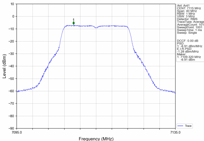
802.11a_HCH_7115MHz_Ant1_NTNV
