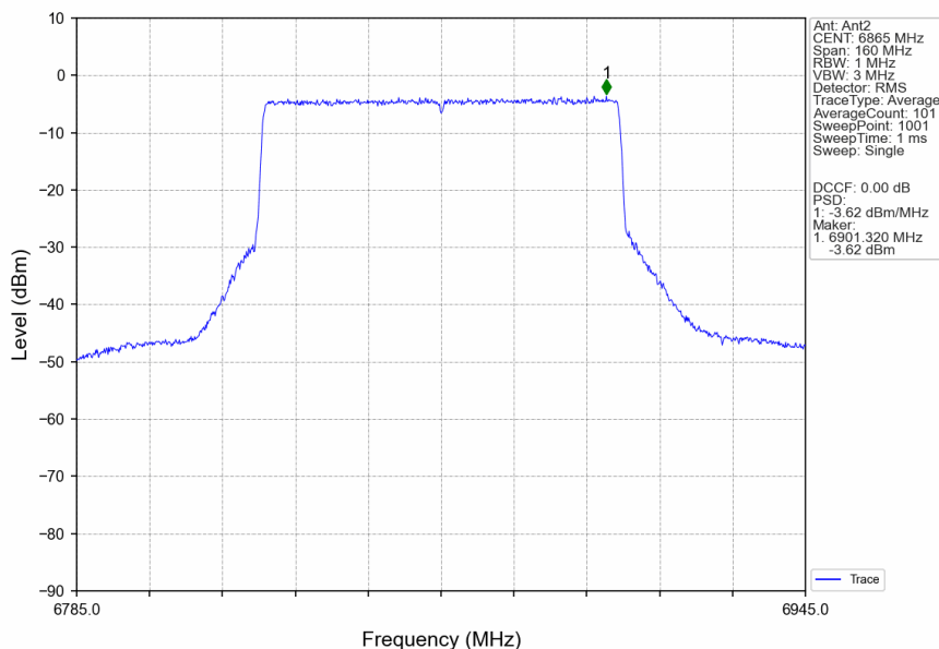
802.11ax(HEW80)_HCH_6865MHz_RU996_Left_Ant2_NTNV
