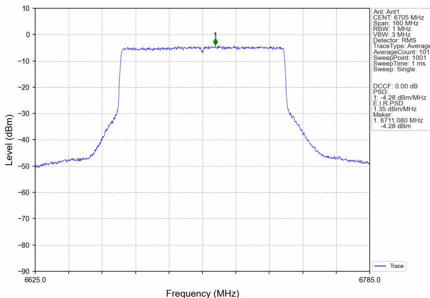
802.11ax(HEW80)_MCH_6705MHz_RU996_Left_Ant1_NTNV
