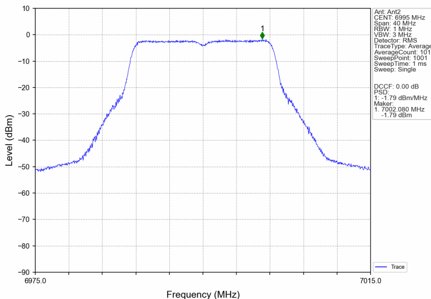
802.11a_MCH_6995MHz_Ant2_NTNV
