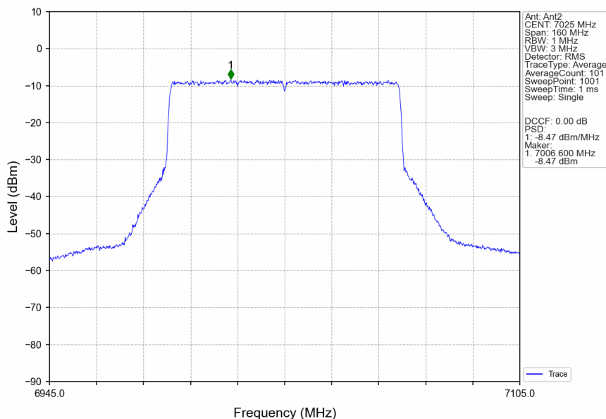
802.11ax(HEW80)_HCH_7025MHz_RU996_Left_Ant2_NTNV
