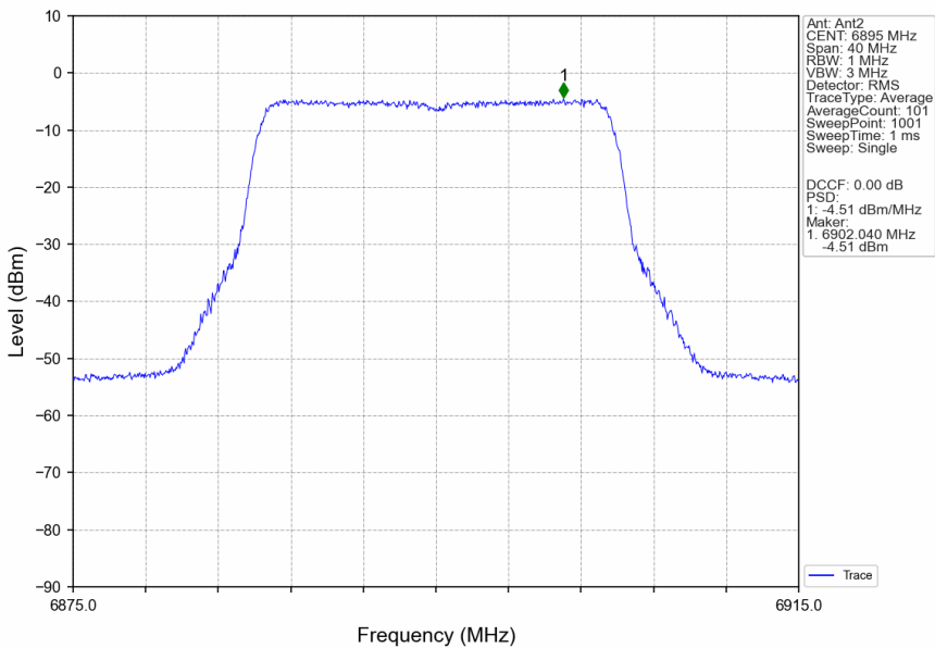
802.11ax(HEW20)_LCH_6895MHz_RU242_Left_Ant2_NTNV
