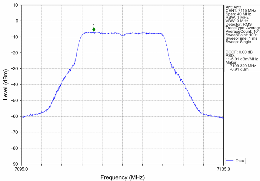
802.11a_HCH_7115MHz_Ant1_NTNV
