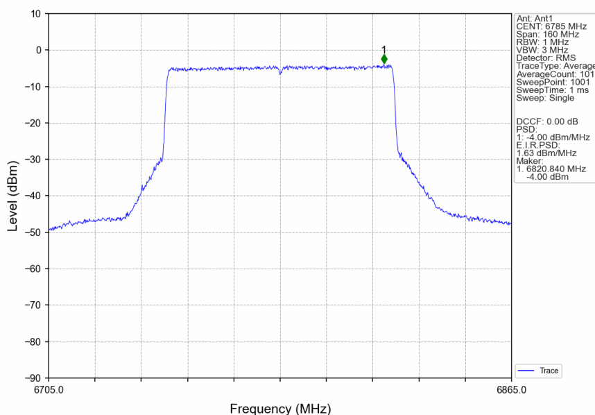
802.11ax(HEW80)_HCH_6785MHz_RU996_Left_Ant1_NTNV
