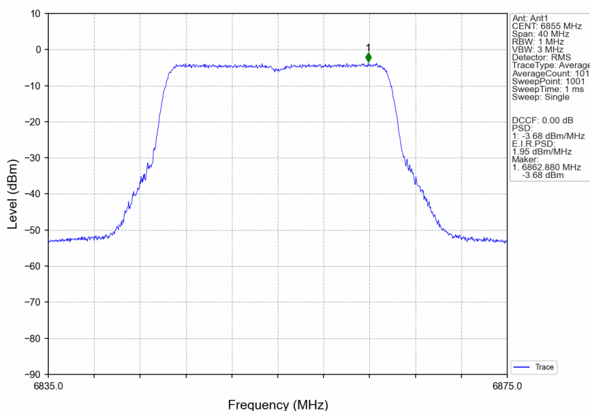
802.11ax(HEW20)_HCH_6855MHz_RU242_Left_Ant1_NTNV
