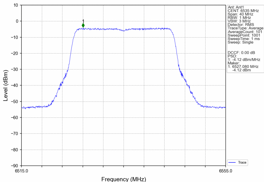
802.11ax(HEW20)_LCH_6535MHz_RU242_Left_Ant1_NTNV
