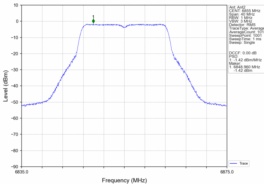
802.11a_HCH_6855MHz_Ant2_NTNV
