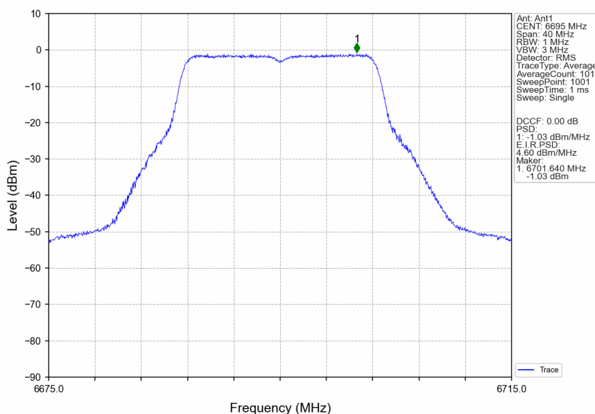
802.11a_MCH_6695MHz_Ant1_NTNV
