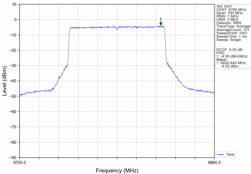
802.11ax(HEW80)_HCH_6785MHz_RU996_Left_Ant1_NTNV
