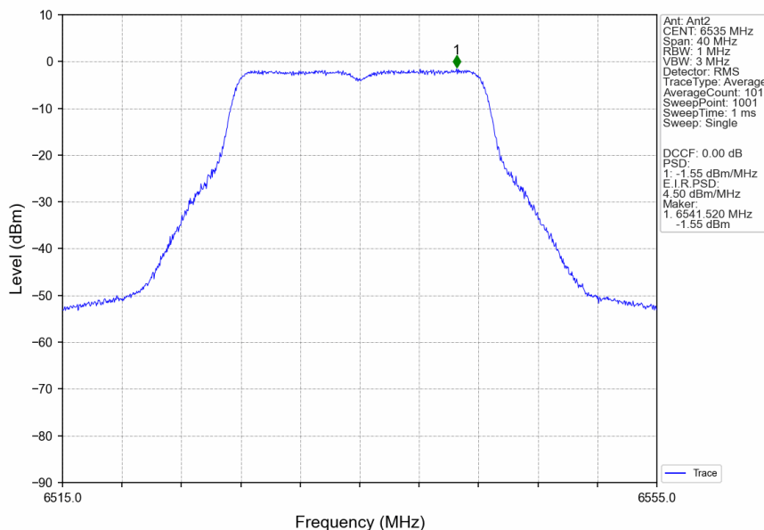
802.11a_LCH_6535MHz_Ant2_NTNV
