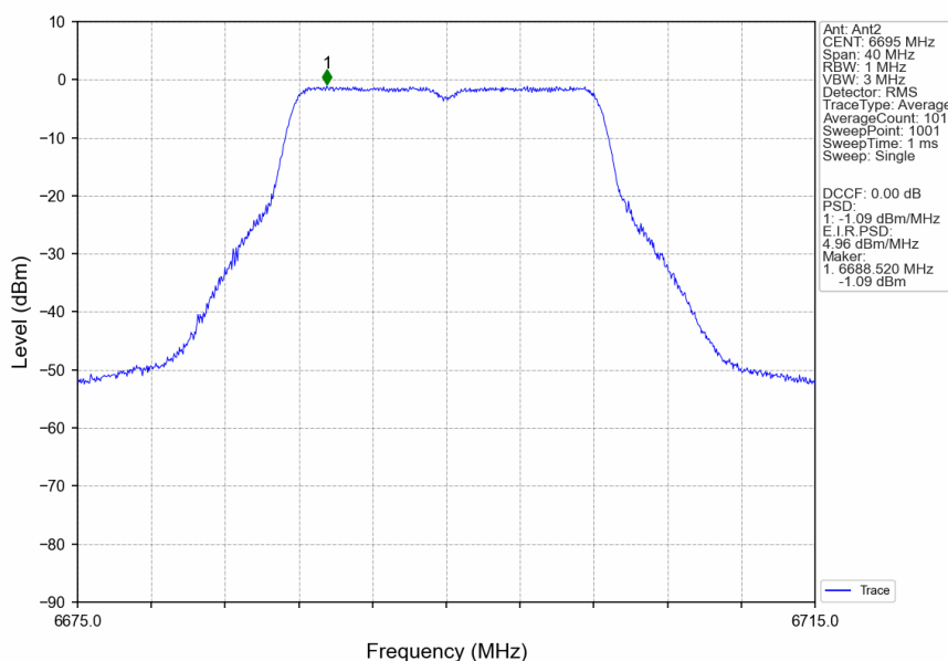
802.11a_MCH_6695MHz_Ant2_NTNV
