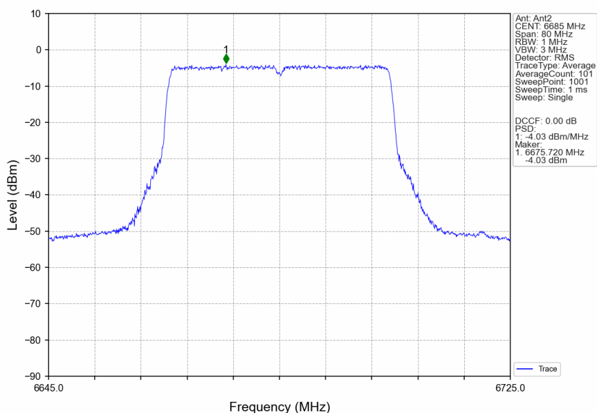
802.11ax(HEW40)_MCH_6685MHz_RU484_Left_Ant2_NTNV
