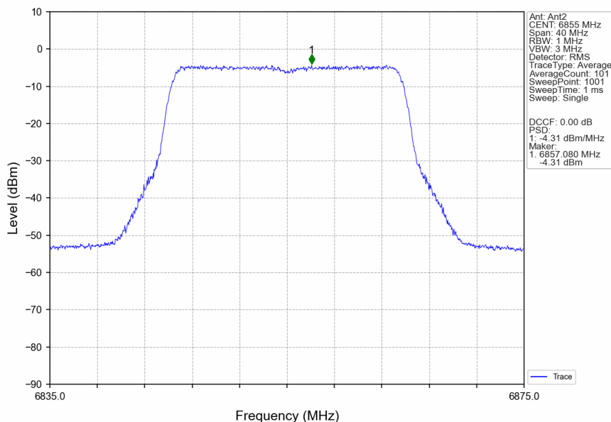
802.11ax(HEW20)_HCH_6855MHz_RU242_Left_Ant2_NTNV
