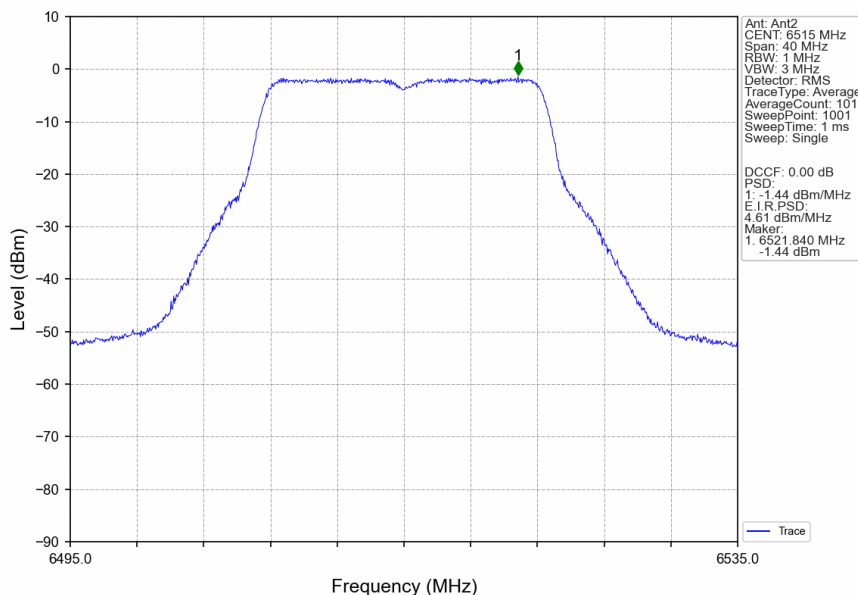
802.11a_HCH_6515MHz_Ant2_NTNV
