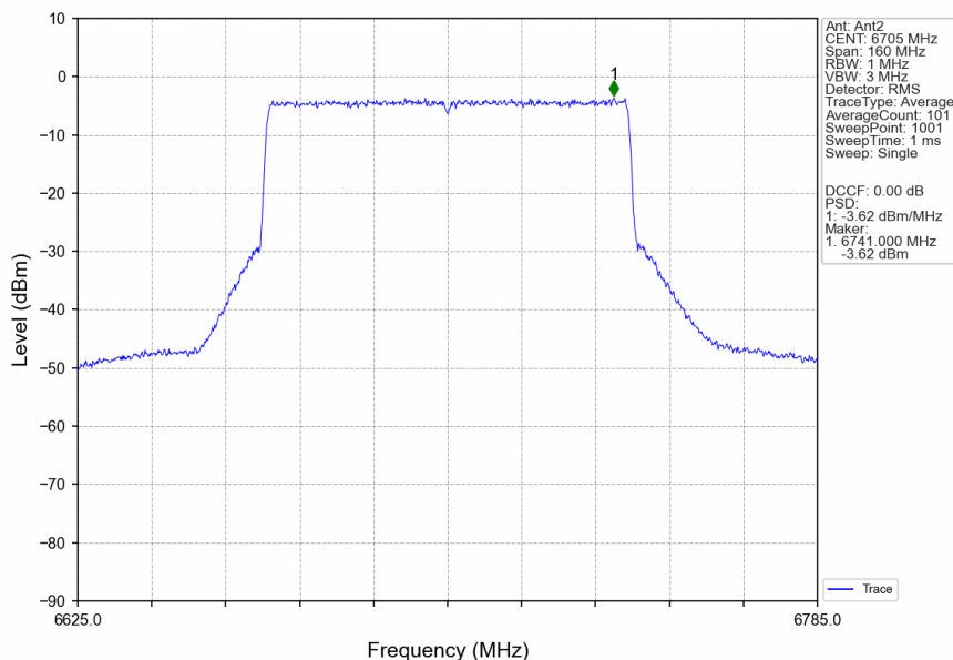
802.11ax(HEW80)_MCH_6705MHz_RU996_Left_Ant2_NTNV
