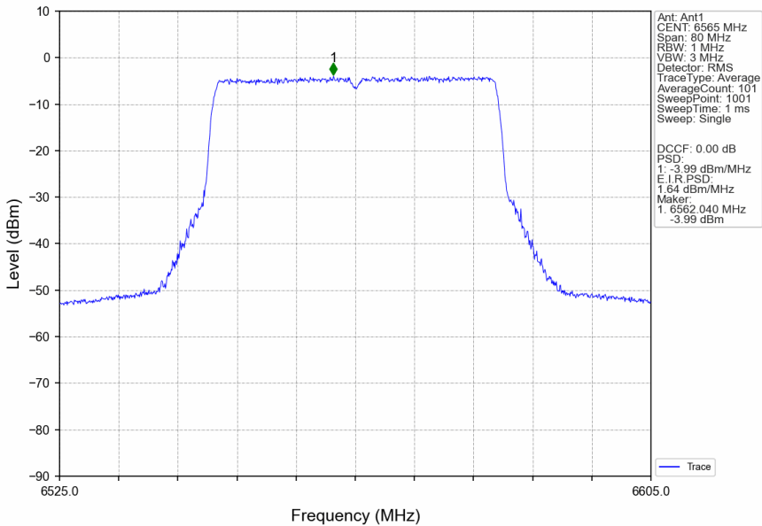
802.11ax(HEW40)_LCH_6565MHz_RU484_Left_Ant1_NTNV
