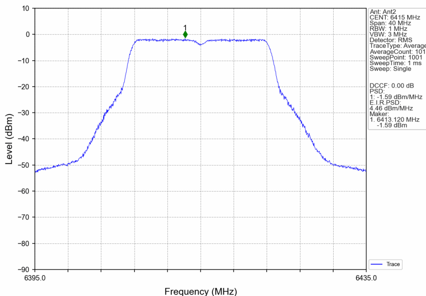
802.11a_HCH_6415MHz_Ant2_NTNV
