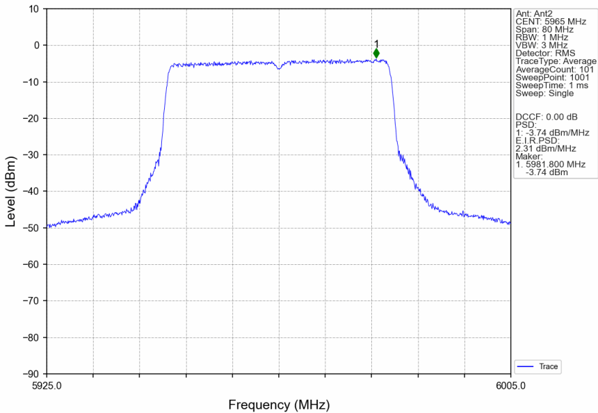
802.11ax(HEW40)_LCH_5965MHz_RU484_Left_Ant2_NTNV
