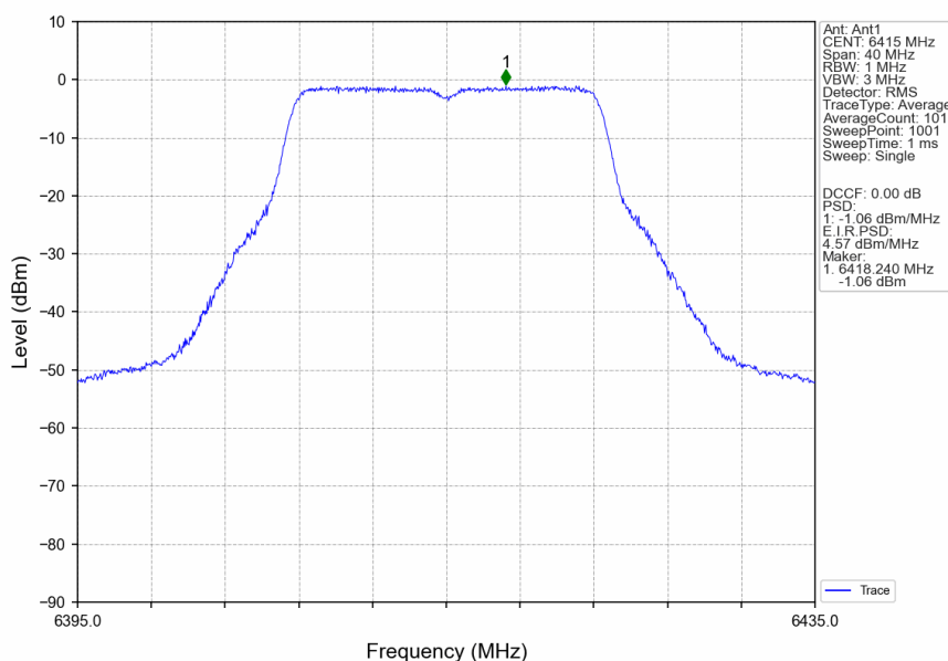
802.11a_HCH_6415MHz_Ant1_NTNV
