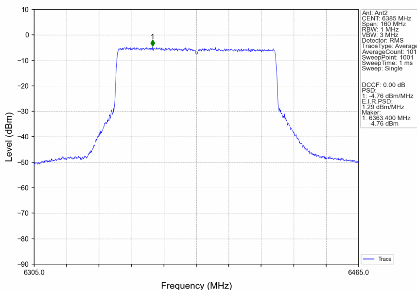
802.11ax(HEW80)_HCH_6385MHz_RU996_Left_Ant2_NTNV
