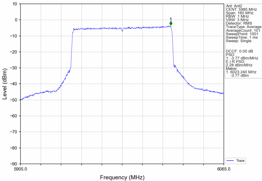
802.11ax(HEW80)_LCH_5985MHz_RU996_Left_Ant2_NTNV
