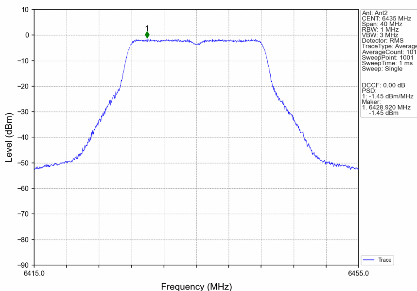
802.11a_LCH_6435MHz_Ant2_NTNV
