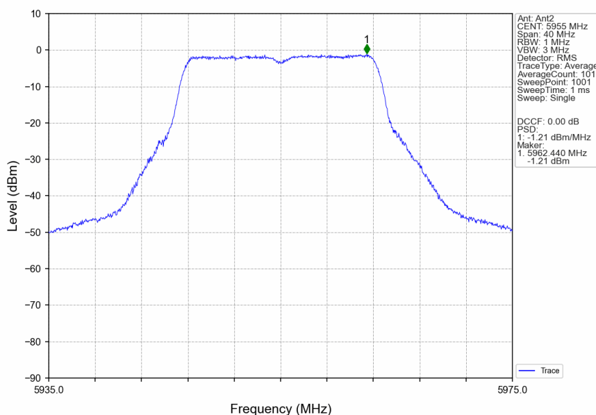
802.11a_LCH_5955MHz_Ant2_NTNV
