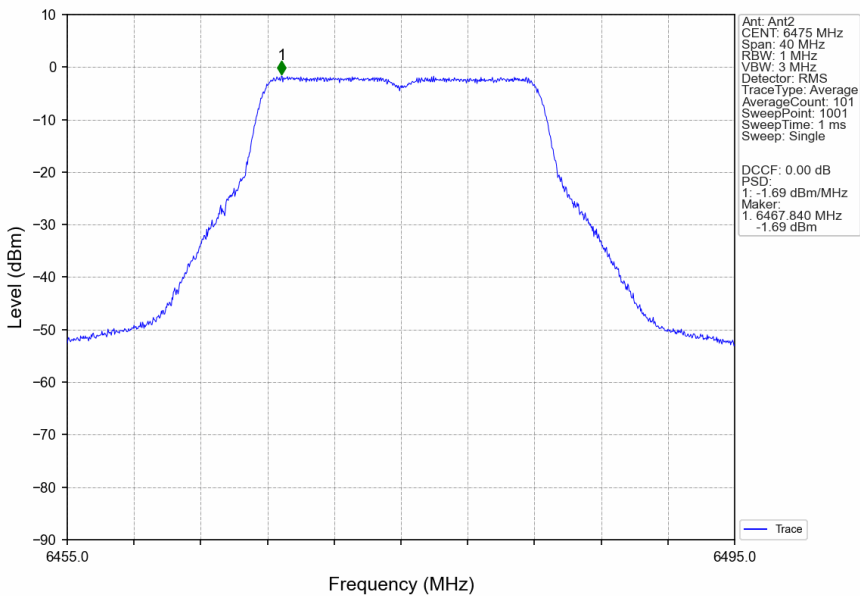
802.11a_MCH_6475MHz_Ant2_NTNV
