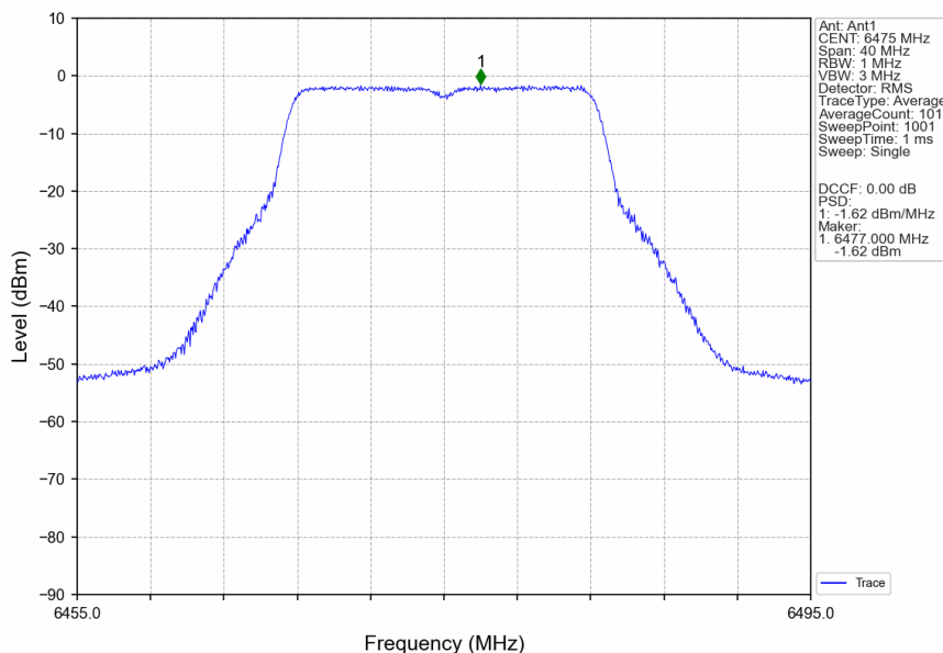
802.11a_MCH_6475MHz_Ant1_NTNV
