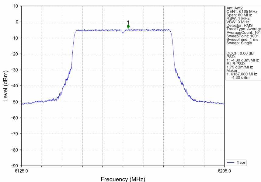
802.11ax(HEW40)_MCH_6165MHz_RU484_Left_Ant2_NTNV
