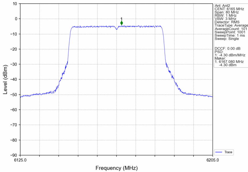
802.11ax(HEW40)_MCH_6165MHz_RU484_Left_Ant2_NTNV
