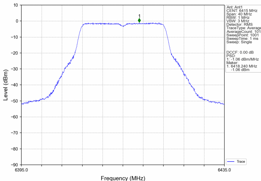
802.11a_HCH_6415MHz_Ant1_NTNV
