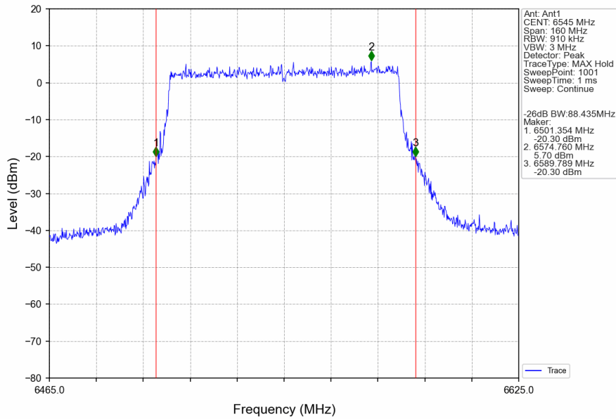
802.11ax(HEW80)_HCH_6545MHz_RU996_Left_Ant1_NTNV
