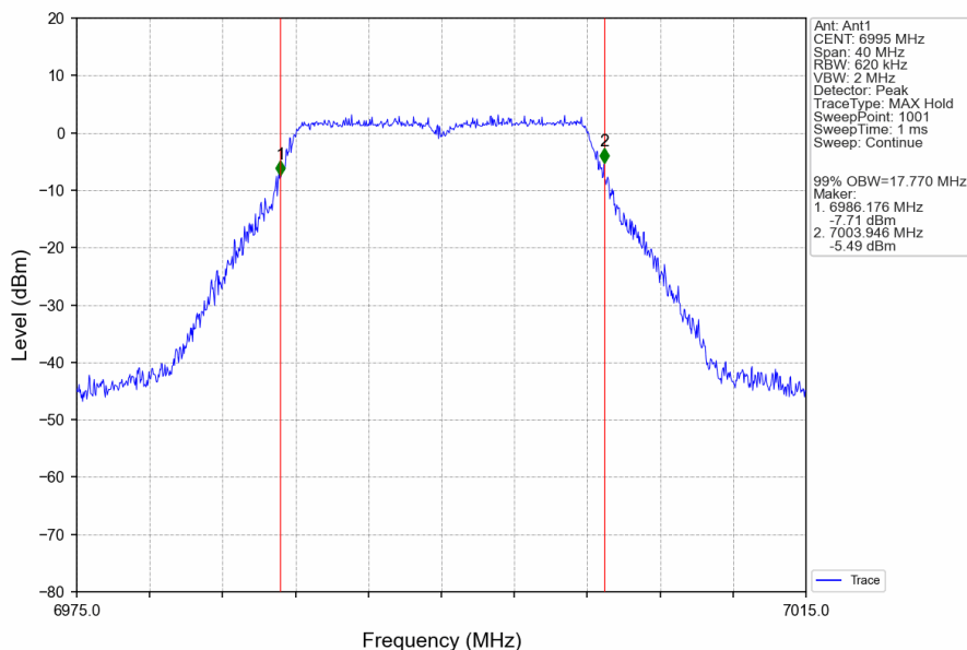
802.11a_MCH_6995MHz_Ant1_NTNV
