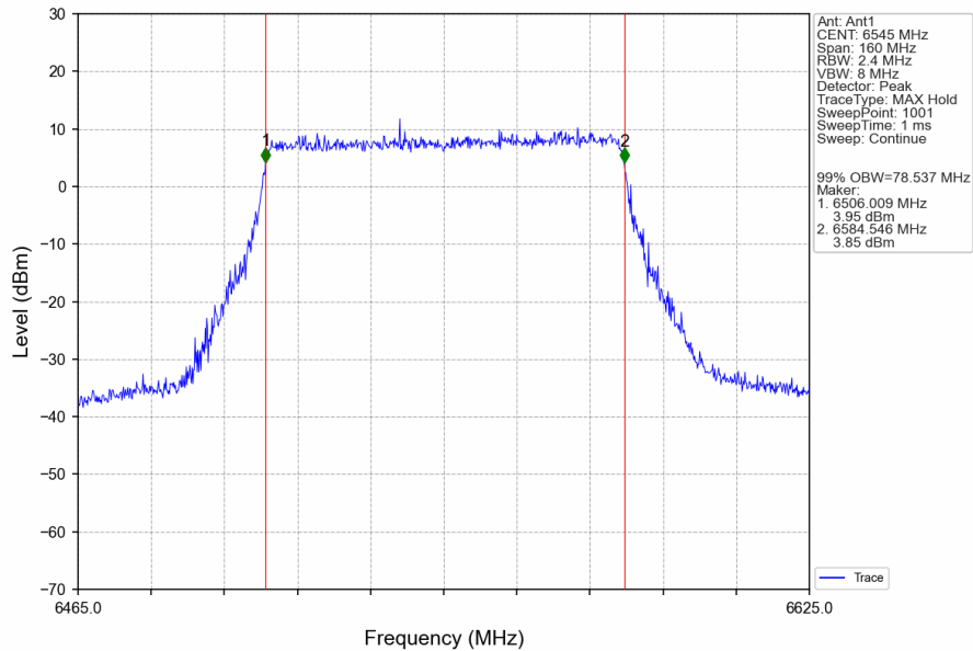
802.11ax(HEW80)_HCH_6545MHz_RU996_Left_Ant1_NTNV
