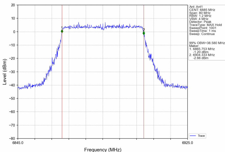
802.11ax(HEW40)_HCH_6885MHz_RU484_Left_Ant1_NTNV
