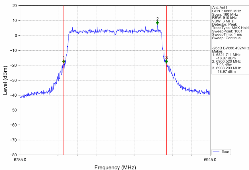
802.11ax(HEW80)_HCH_6865MHz_RU996_Left_Ant1_NTNV
