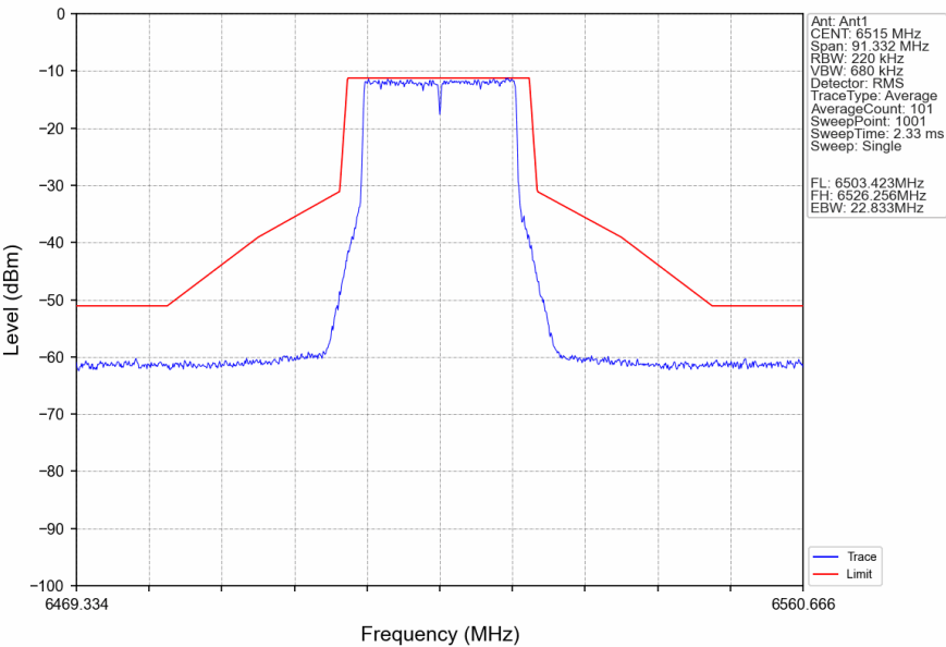
802.11be(EHT20)_HCH_6515MHz_RU242_Left_Ant1_NTNV
