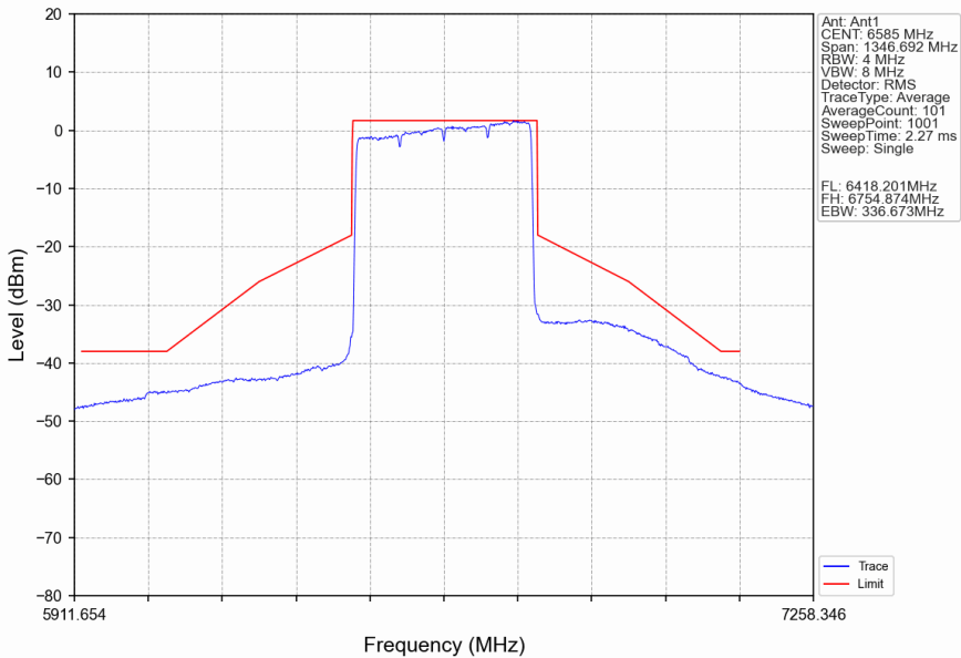
802.11be(EHT320)_MCH_6585MHz_4xRU996_Left_Ant1_NTNV
