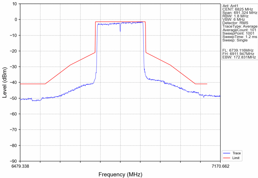
802.11be(EHT160)_HCH_6825MHz_2xRU996_Left_Ant1_NTNV
