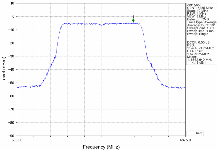
802.11be(EHT20)_HCH_6855MHz_RU242_Left_Ant2_NTNV
