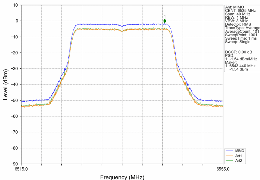
802.11be(EHT20)_LCH_6535MHz_RU242_Left_MIMO_NTNV
