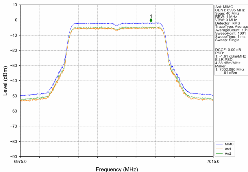
802.11be(EHT20)_MCH_6995MHz_RU242_Left_MIMO_NTNV
