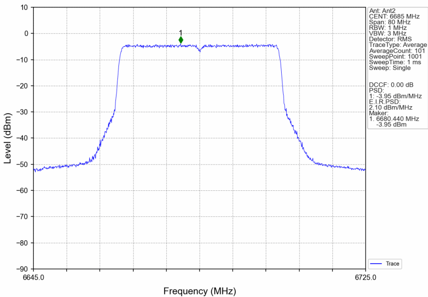
802.11be(EHT40)_MCH_6685MHz_RU484_Left_Ant2_NTNV
