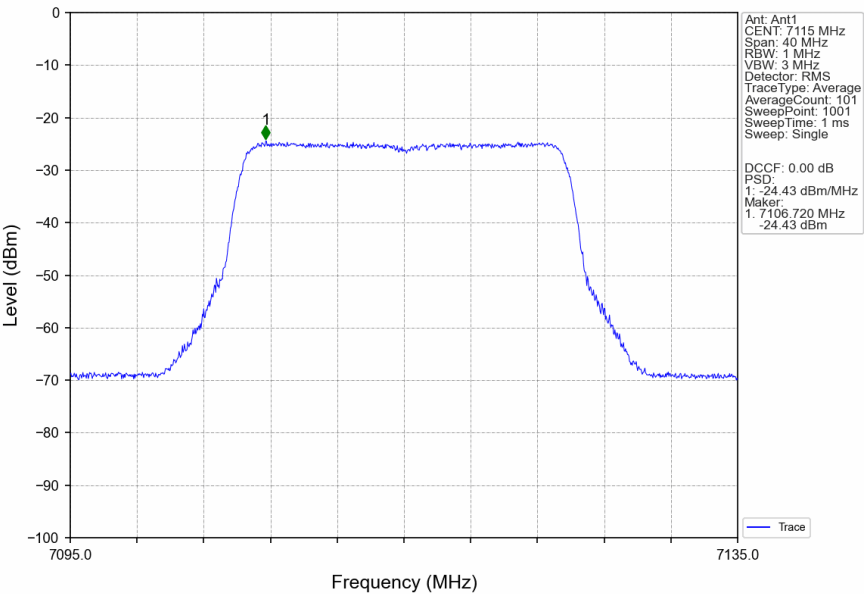
802.11be(EHT20)_HCH_7115MHz_RU242_Left_Ant1_NTNV
