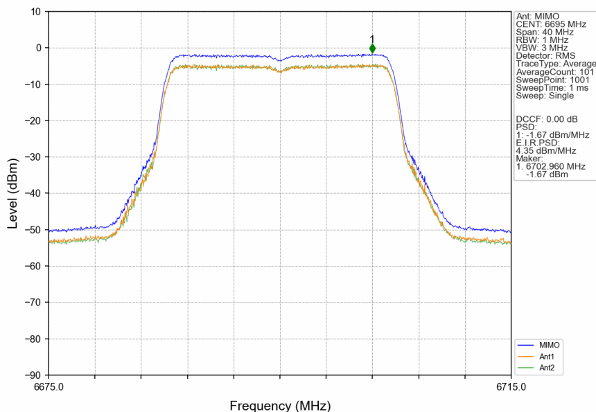
802.11be(EHT20)_MCH_6695MHz_RU242_Left_MIMO_NTNV
