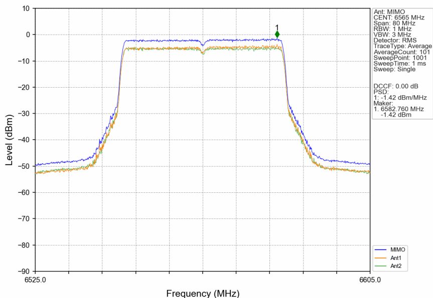
802.11be(EHT40)_LCH_6565MHz_RU484_Left_MIMO_NTNV
