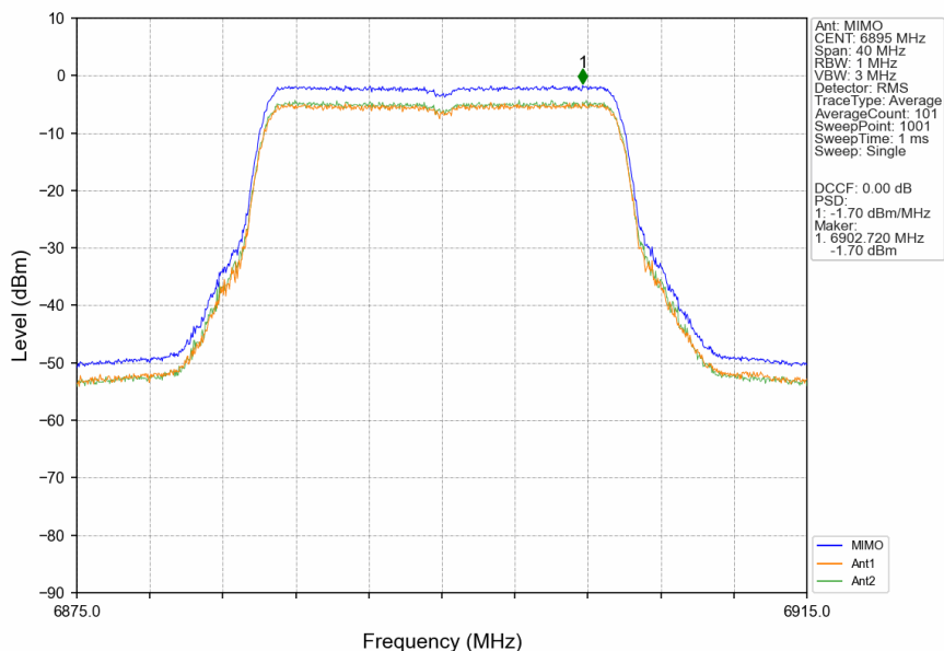
802.11be(EHT20)_LCH_6895MHz_RU242_Left_MIMO_NTNV
