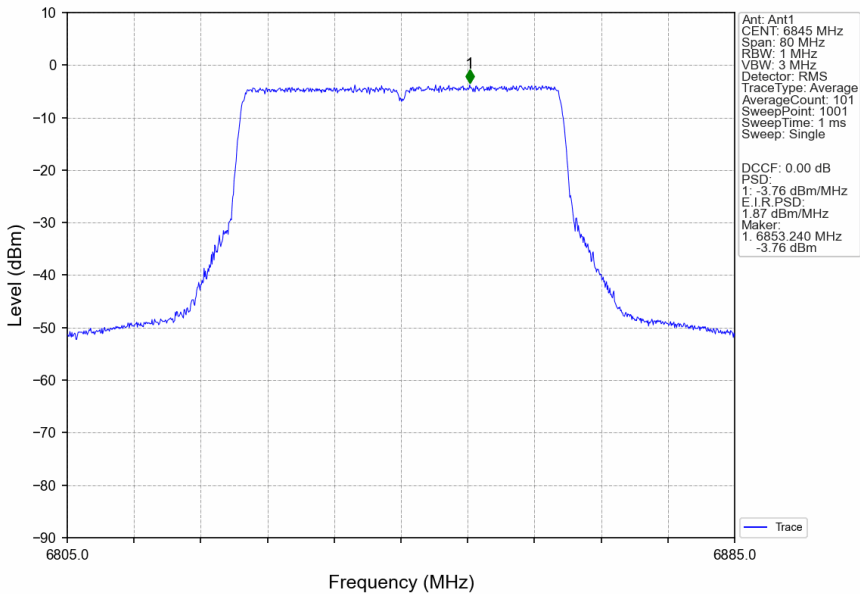
802.11be(EHT40)_HCH_6845MHz_RU484_Left_Ant1_NTNV
