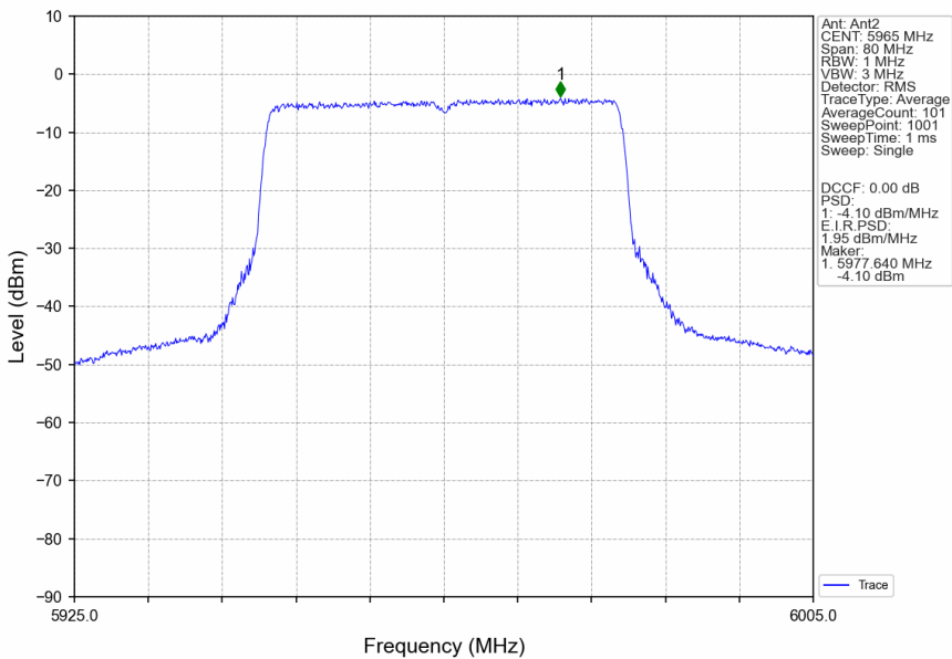
802.11be(EHT40)_LCH_5965MHz_RU484_Left_Ant2_NTNV
