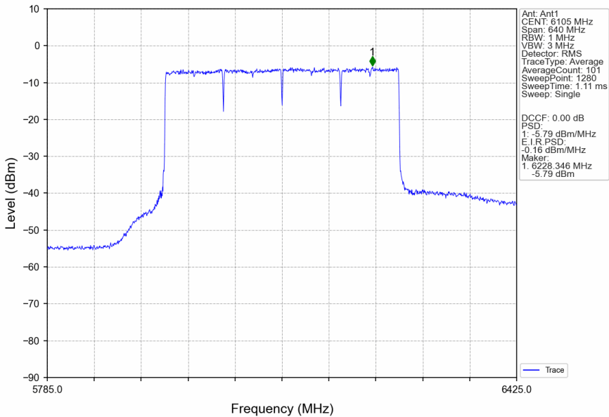
802.11be(EHT320)_LCH_6105MHz_4xRU996_Left_Ant1_NTNV
