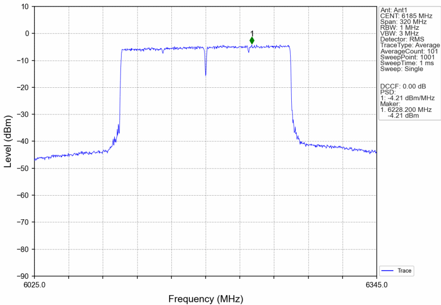
802.11be(EHT160)_MCH_6185MHz_2xRU996_Left_Ant1_NTNV
