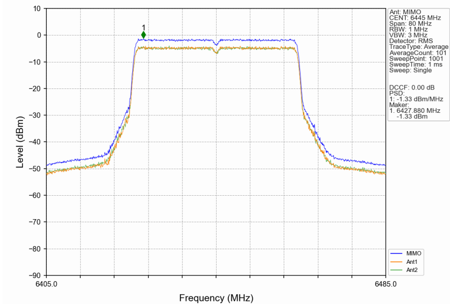
802.11be(EHT40)_LCH_6445MHz_RU484_Left_MIMO_NTNV
