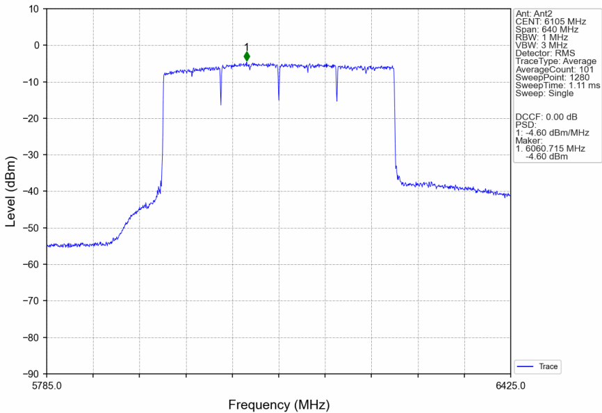
802.11be(EHT320)_LCH_6105MHz_4xRU996_Left_Ant2_NTNV
