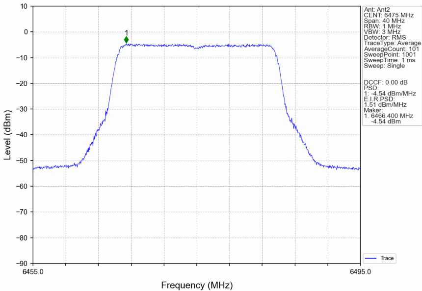
802.11be(EHT20)_MCH_6475MHz_RU242_Left_Ant2_NTNV
