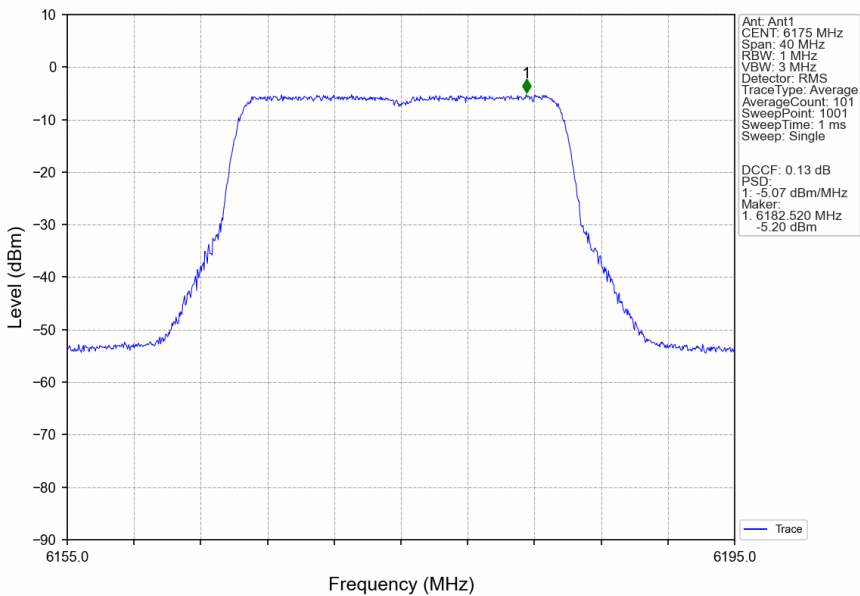
802.11be(EHT20)_MCH_6175MHz_RU242_Left_Ant1_NTNV
