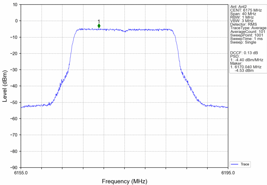
802.11be(EHT20)_MCH_6175MHz_RU242_Left_Ant2_NTNV
