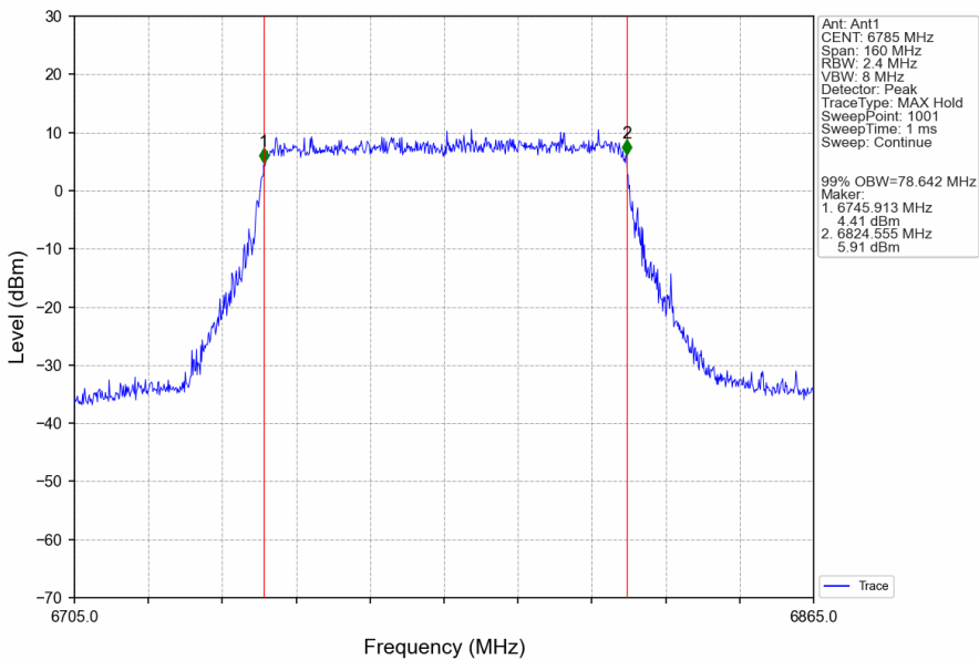
802.11be(EHT80)_HCH_6785MHz_RU996_Left_Ant1_NTNV
