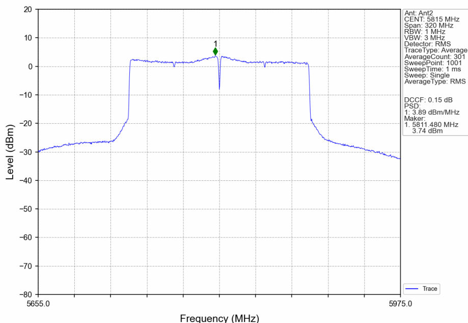
802.11be(EHT160)_HCH_5815MHz_SU_ / _MIMO_NTNV
