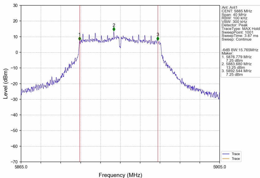
802.11a_HCH_5885MHz_Ant1_NTNV
