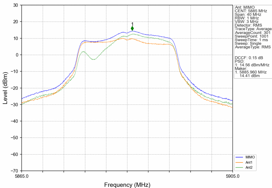
802.11n(HT20)_HCH_5885MHz_MIMO_NTNV
