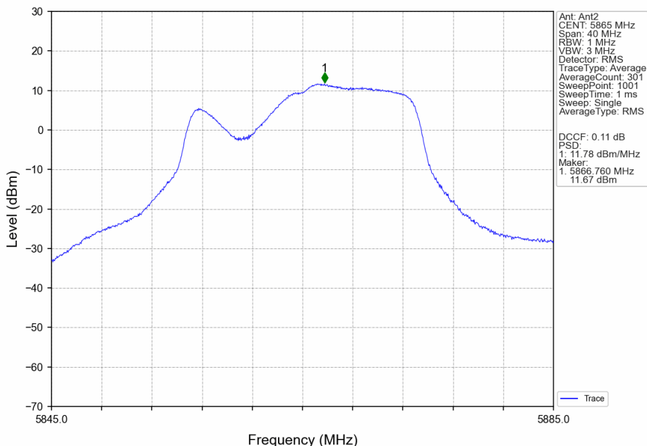
802.11ac(VHT20)_LCH_5865MHz_MIMO_NTNV
