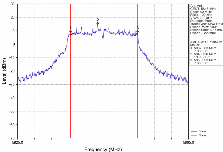
802.11a_HCH_5845MHz_Ant1_NTNV
