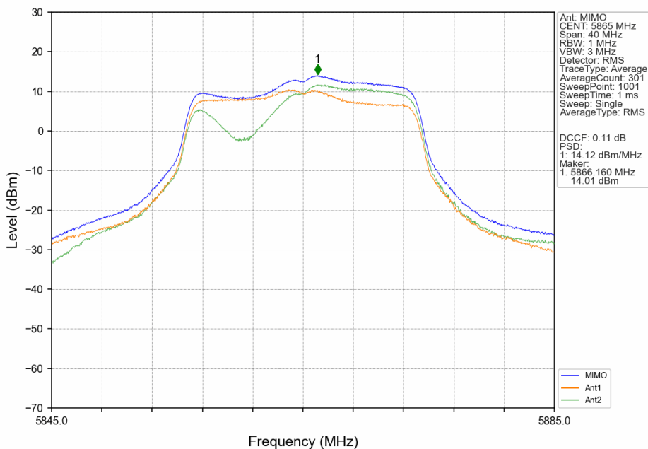
802.11ac(VHT20)_LCH_5865MHz_MIMO_NTNV
