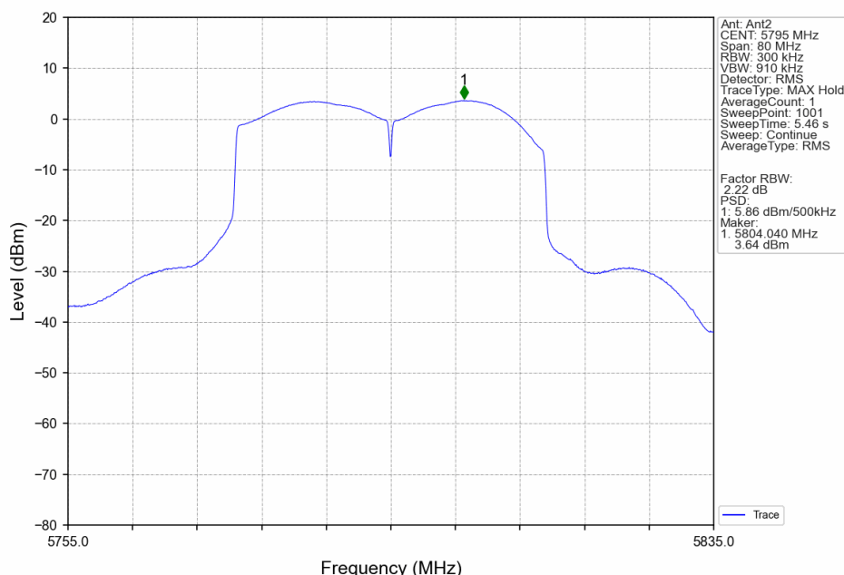
802.11be(EHT40)_HCH_5795MHz_SU_ / _Ant2_NTNV
