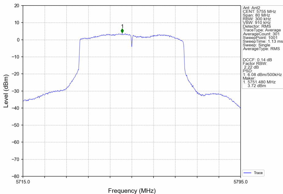
802.11be(EHT40)_LCH_5755MHz_SU_ / _MIMO_NTNV
