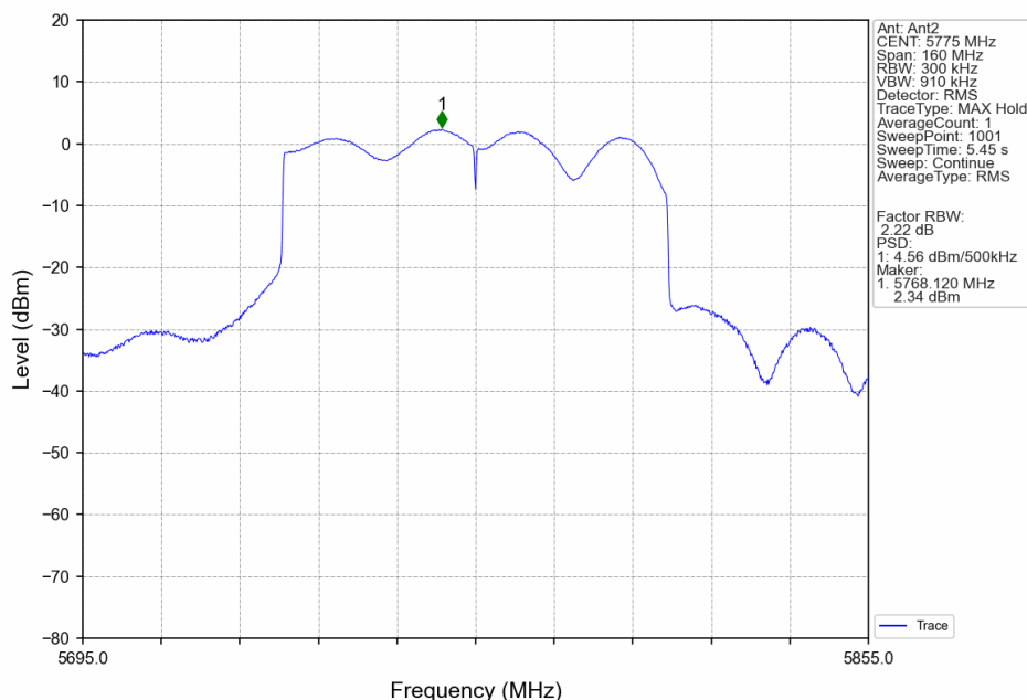
802.11ax(HEW80)_MCH_5775MHz_SU_ / _MIMO_NTNV
