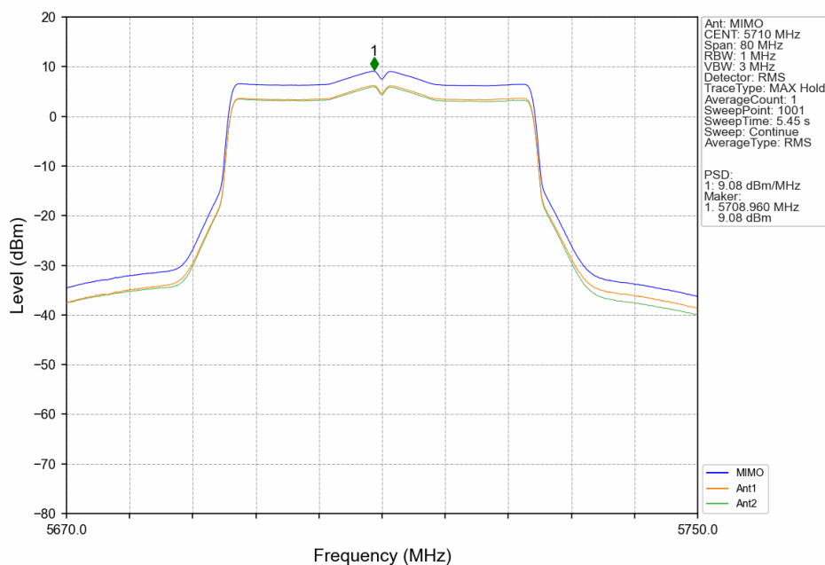
802.11be(EHT40)_HCH_5710MHz_SU_ / _MIMO_NTNV
