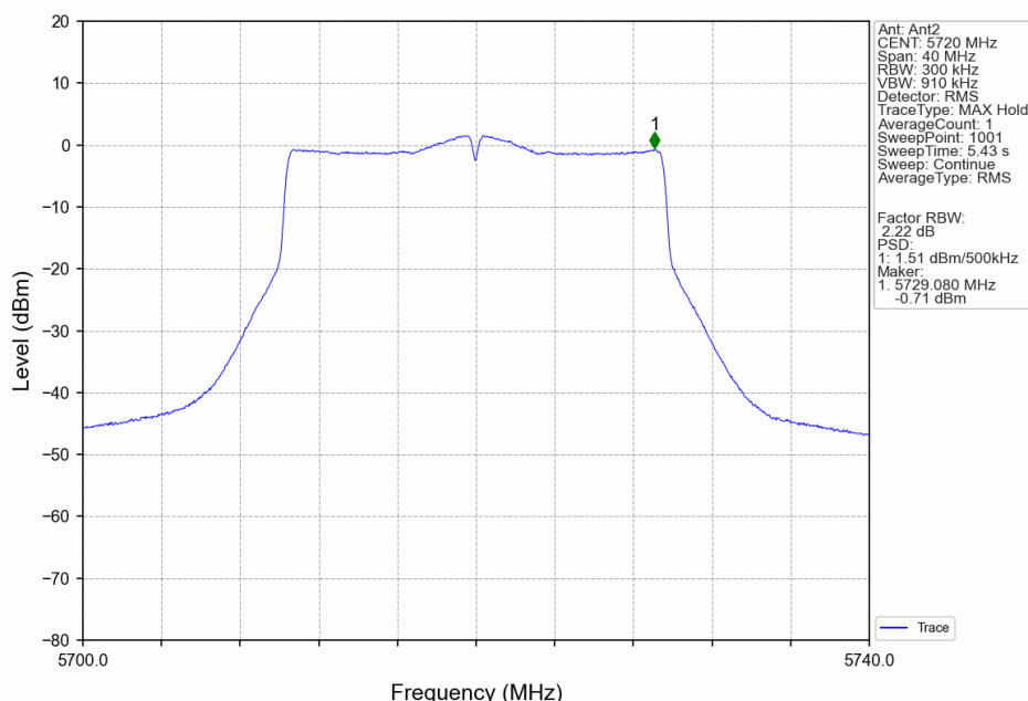
802.11ac(VHT20)_HCH_5720MHz_Ant2_NTNV
