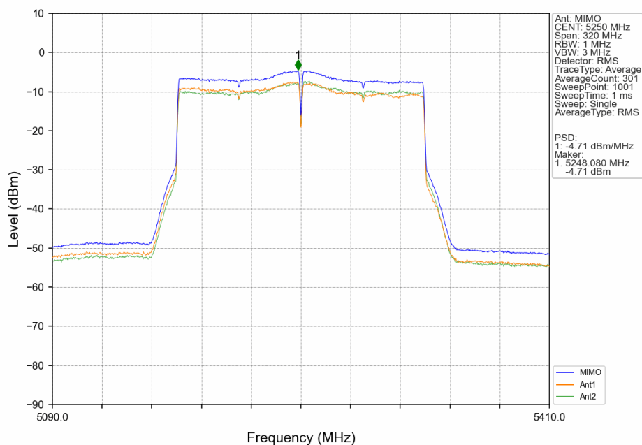
802.11be(EHT160)_MCH_5250MHz_SU_ / _MIMO_NTNV
