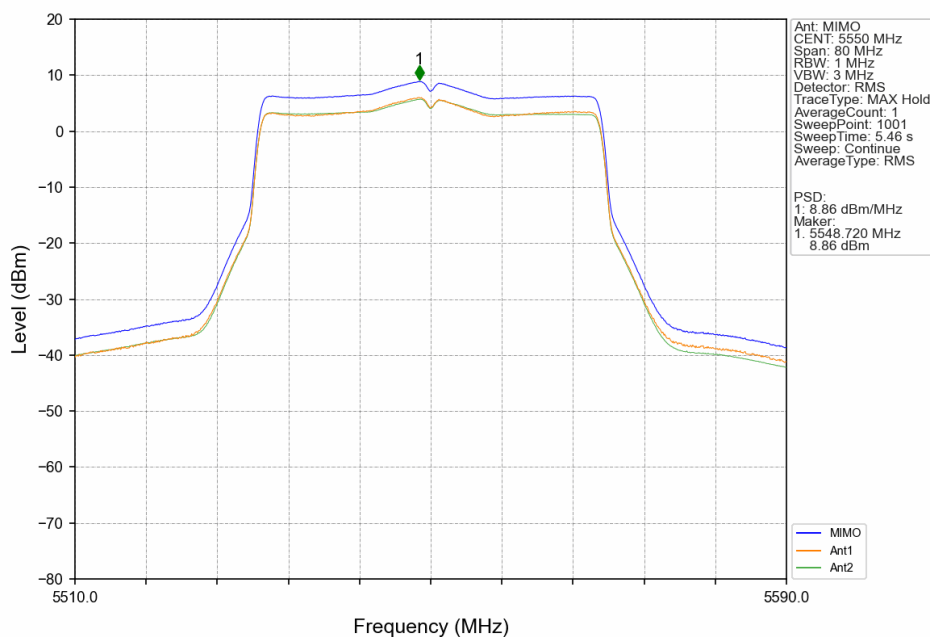
802.11be(EHT40)_MCH_5550MHz_SU_ / _MIMO_NTNV
