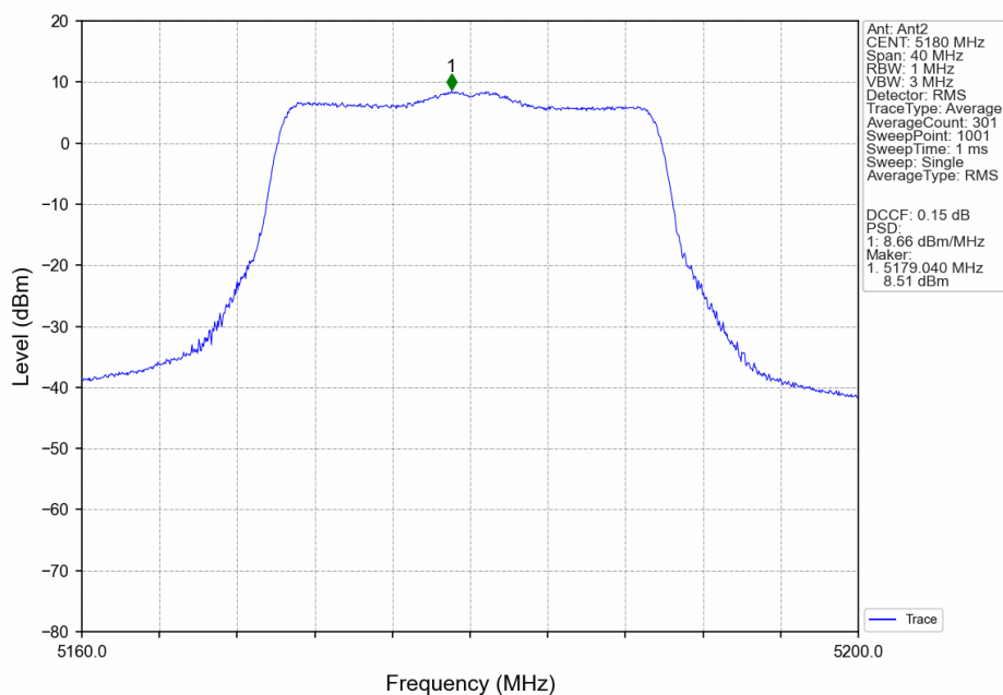
802.11be(EHT20)_LCH_5180MHz_SU_ / _Ant2_NTNV
