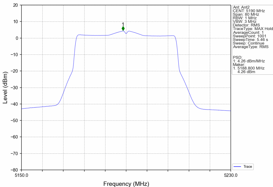
802.11be(EHT40)_LCH_5190MHz_SU_ / _Ant2_NTNV
