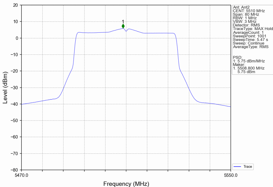
802.11be(EHT40)_LCH_5510MHz_SU_ / _Ant2_NTNV
