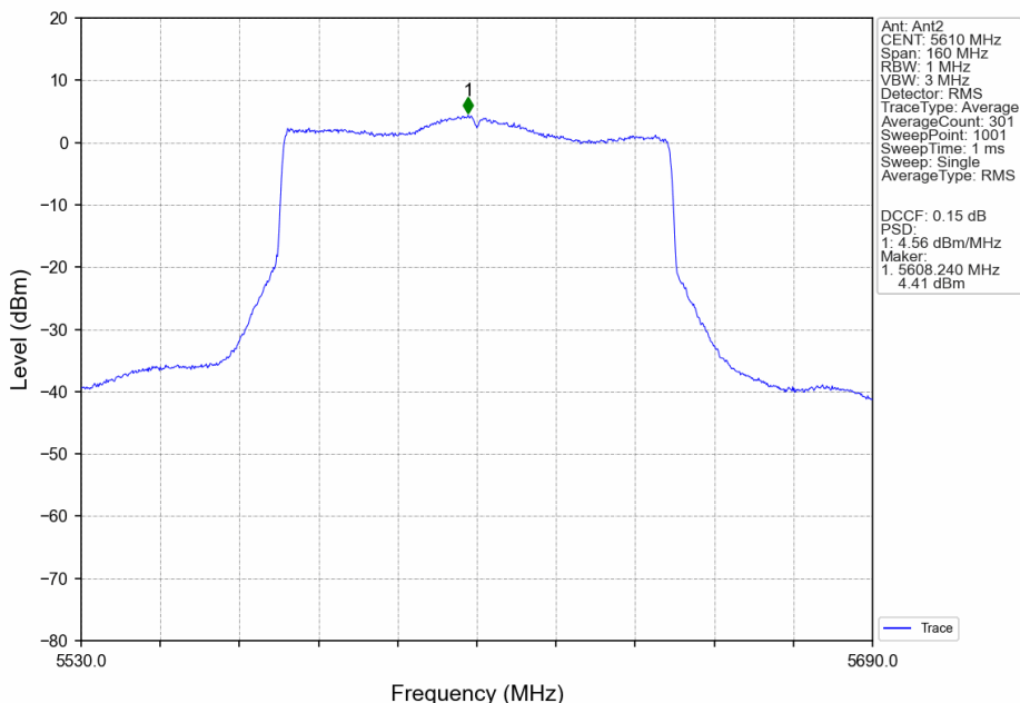
802.11ax(HEW80)_HCH_5610MHz_SU_/_MIMO_NTNV
