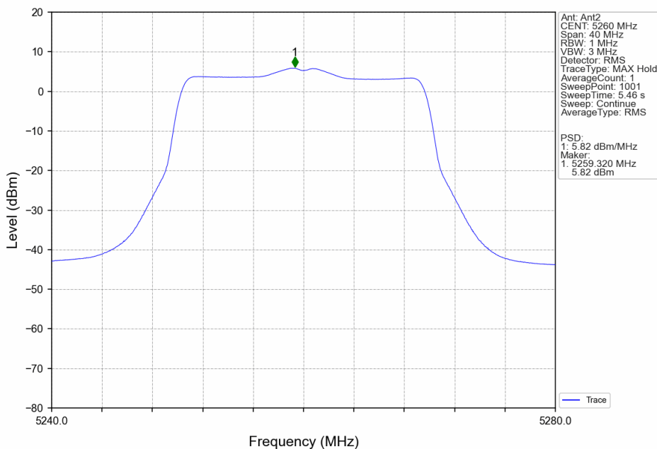
802.11be(EHT20)_LCH_5260MHz_SU_ / _Ant2_NTNV
