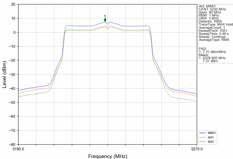
802.11be(EHT40)_HCH_5230MHz_SU_ / _MIMO_NTNV
