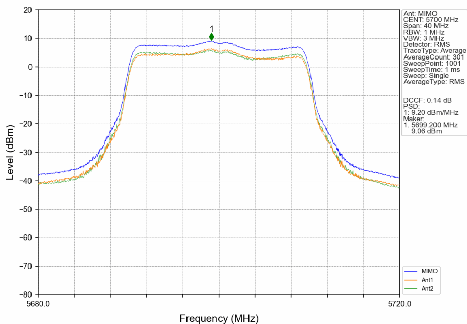
802.11be(EHT20)_HCH_5700MHz_SU_ / _MIMO_NTNV
