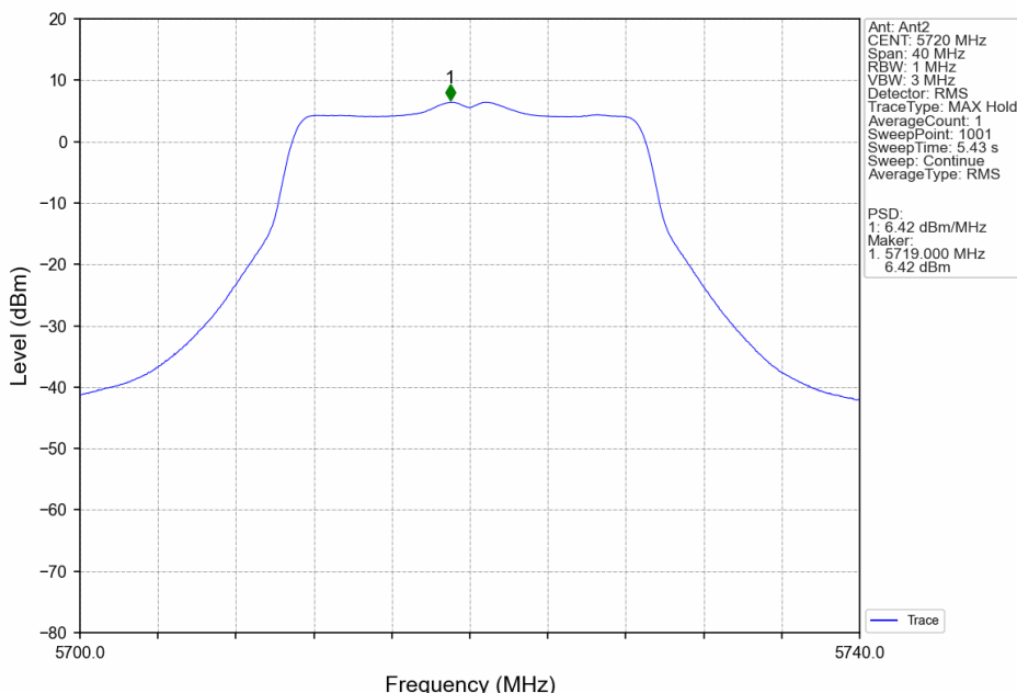
802.11ac(VHT20)_HCH_5720MHz_Ant2_NTNV
