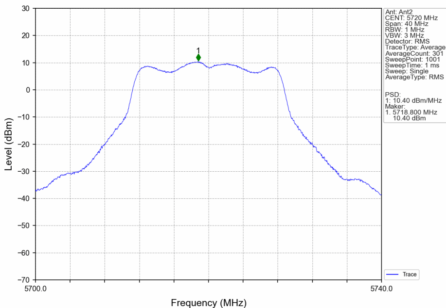
802.11a_HCH_5720MHz_Ant2_NTNV
