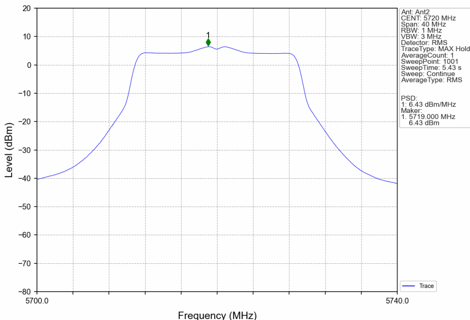
802.11n(HT20)_HCH_5720MHz_MIMO_NTNV
