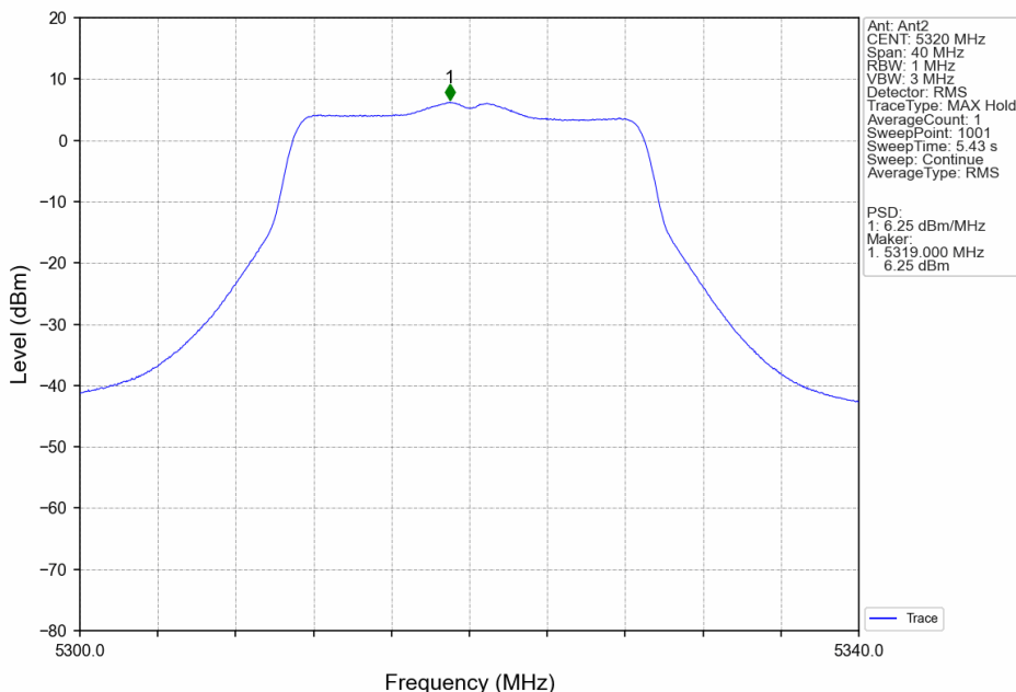
802.11n(HT20)_HCH_5320MHz_MIMO_NTNV
