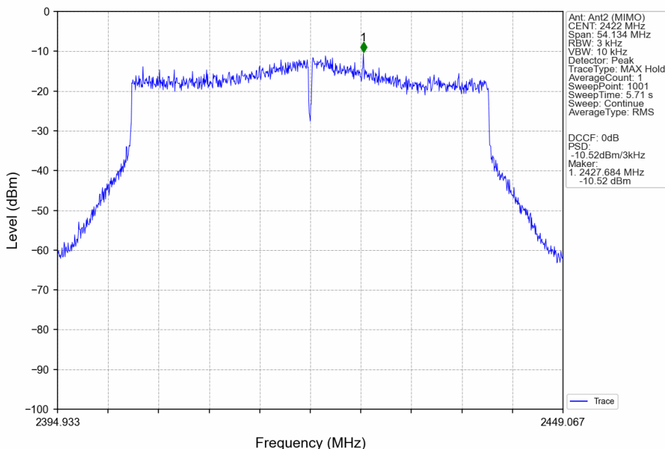
802.11be(EHT40)_LCH_2422MHz_SU_/_MIMO_NTNV
