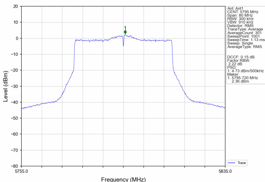
802.11be(EHT40)_HCH_5795MHz_SU_ / _Ant1_NTNV
