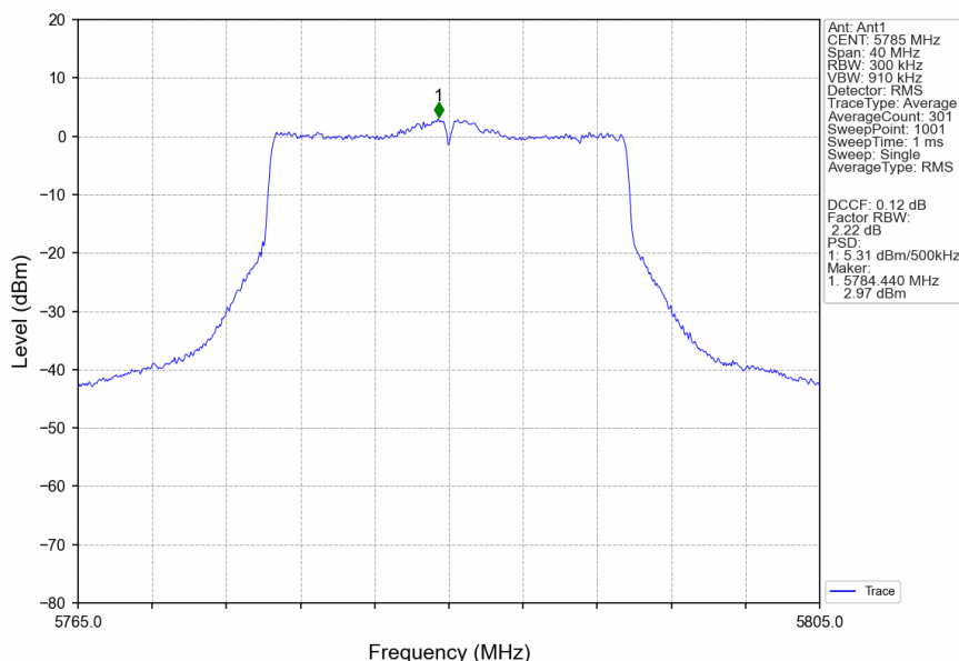
802.11be(EHT20)_MCH_5785MHz_SU_ / _Ant1_NTNV
