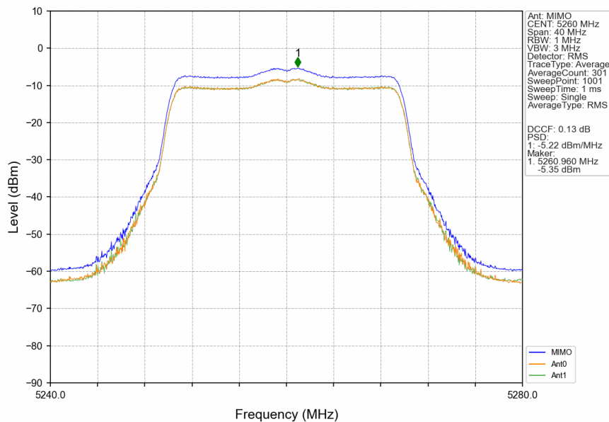
802.11be(EHT20)_LCH_5260MHz_SU_ / _MIMO_NTNV
