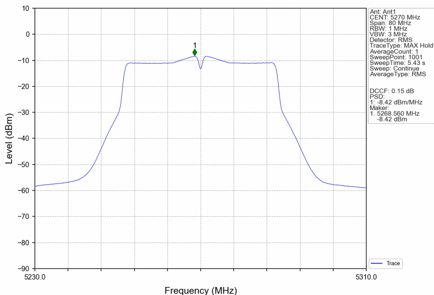
802.11n(HT40)_LCH_5270MHz_MIMO_NTNV
